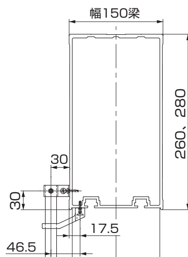
梁260、280の場合
