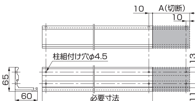
図3-2 根太掛け（後側） 片側切詰めの場合
