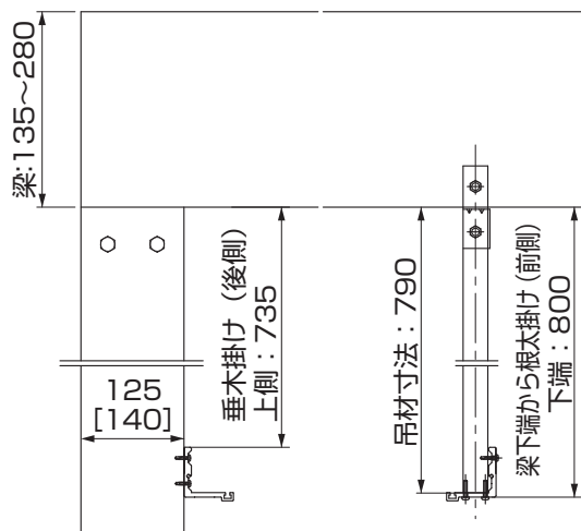
図5-1 正面図
