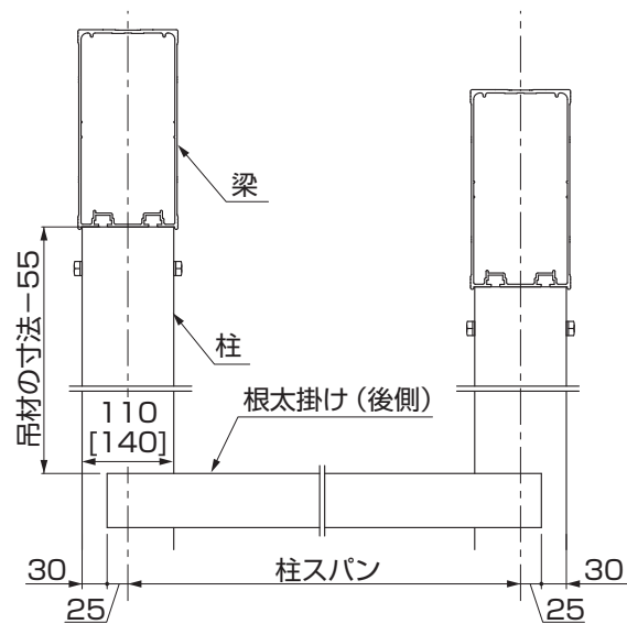
図5-2 側面図
