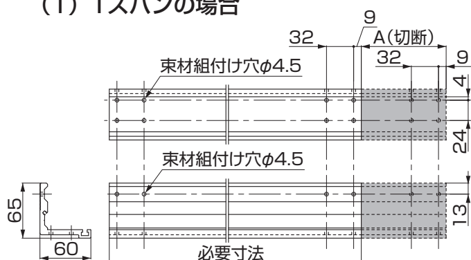
図3-1 根太掛け（前側） 片側切詰めの場合
