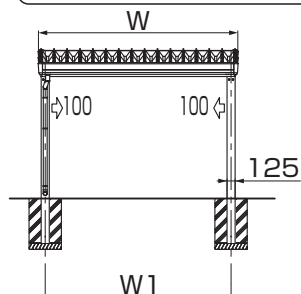
図2-1 間口30・36サイズ
