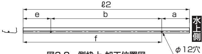
図3-2 側枠上 加工位置図
