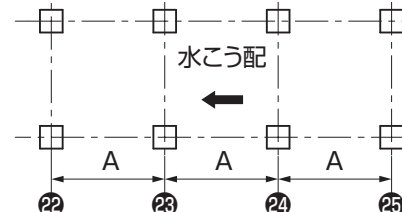
図1-5 6本柱+12延長
