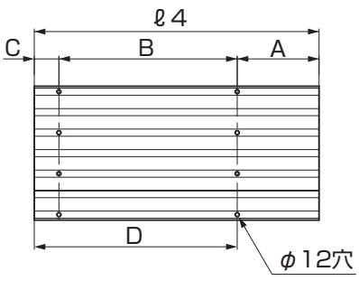
図3-4 折板上 加工位置図
