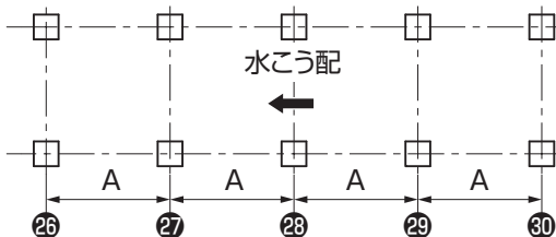
図1-6 8本柱+12延長
