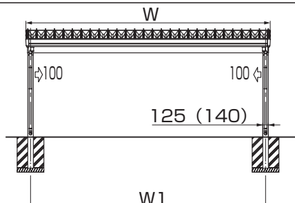
図2-2 間口48・55・60サイズ
