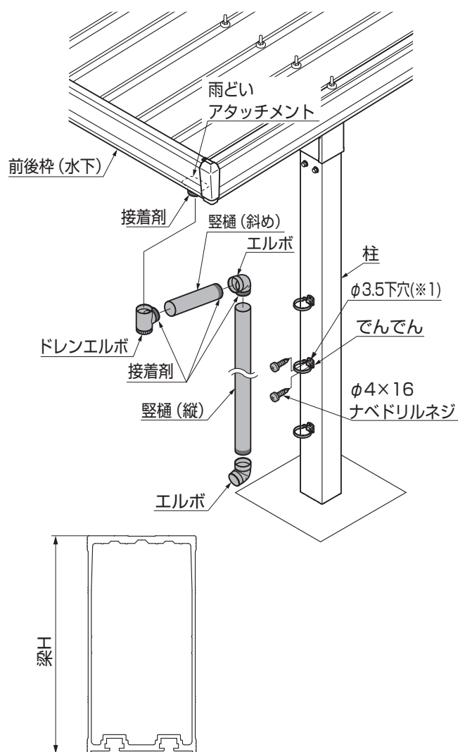
図7-1 梁高さH
