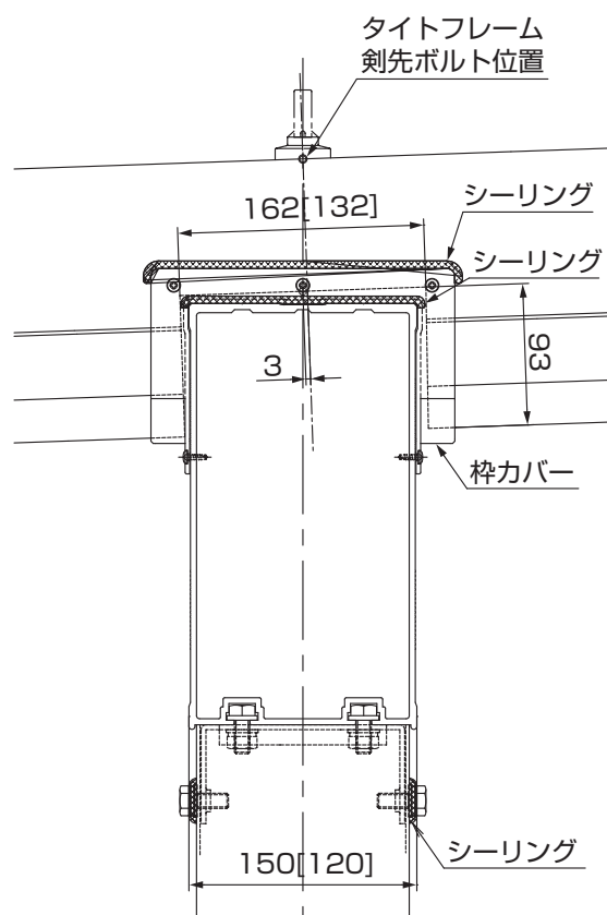
図1-1 梁幅150の場合 (梁260、280) ※ [ ]内は梁幅120の場合 (梁135、200、240)
