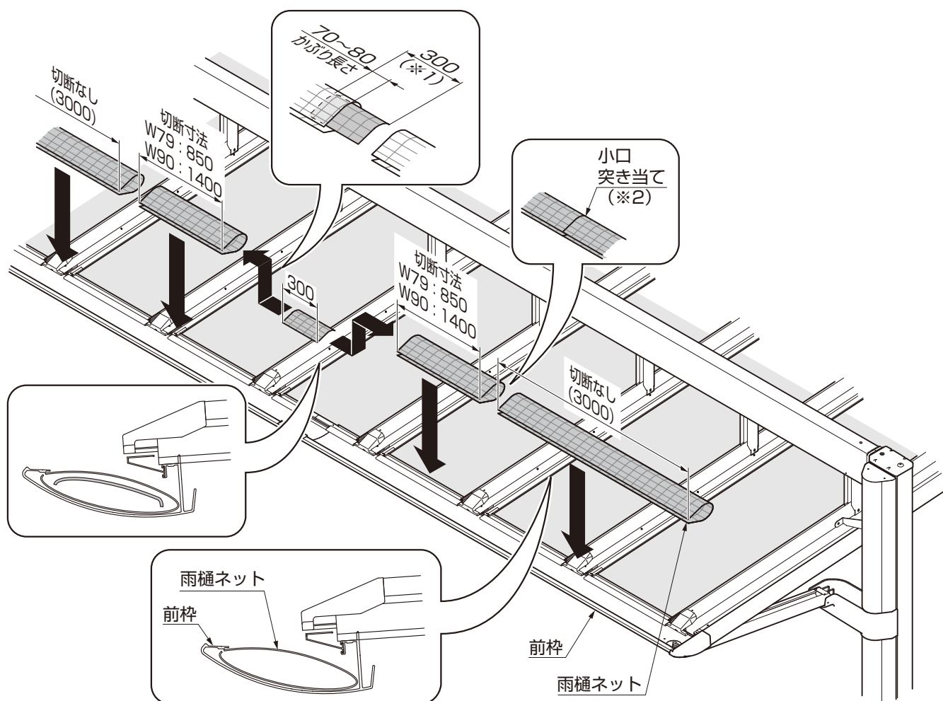
図1-2 雨樋ネット切断寸法（1枚を切断してください。）
