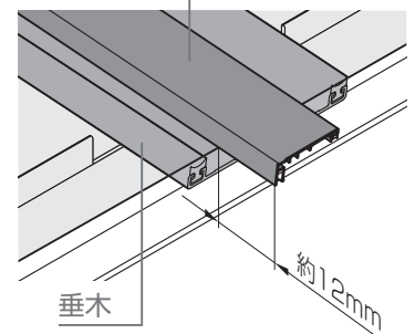
垂木カバー
