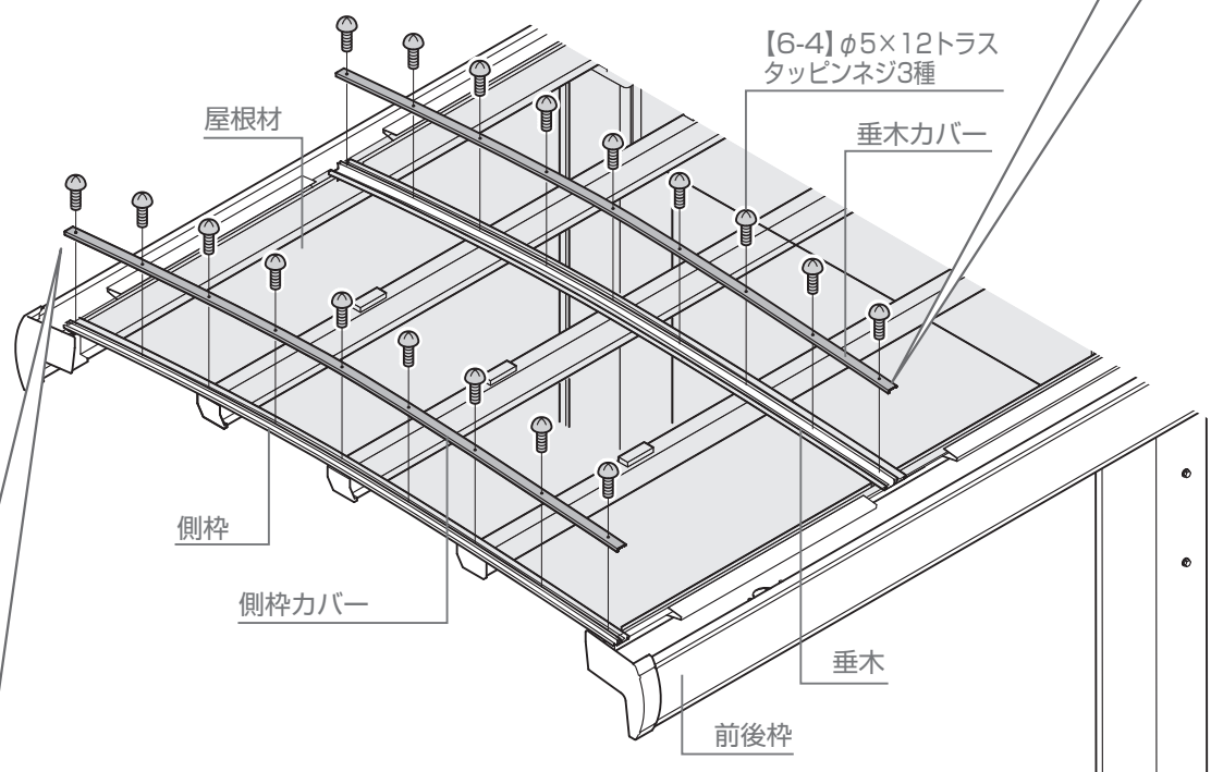
前後枠
