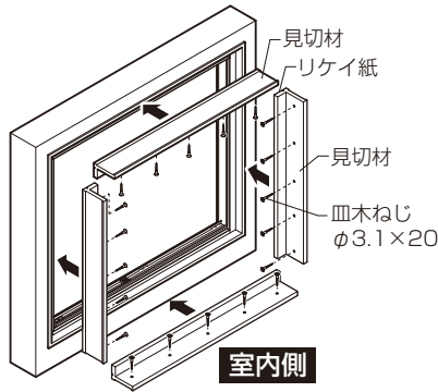
FIX側
