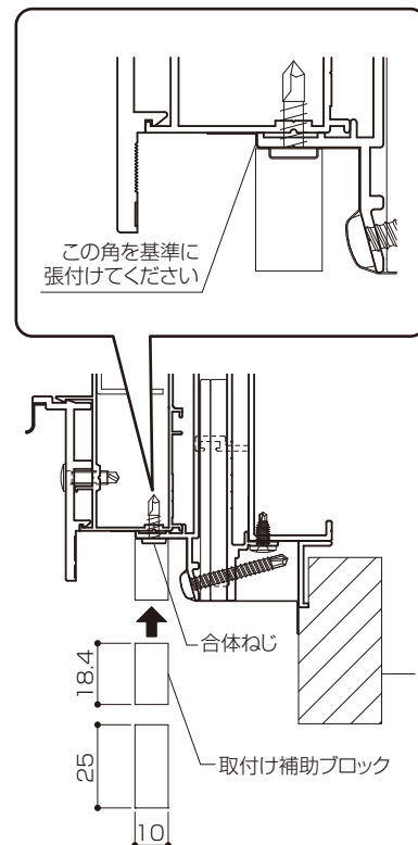
●縦断面図
