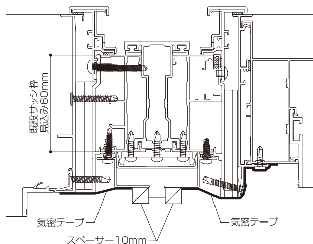
連窓方立カバー受け材の場合
