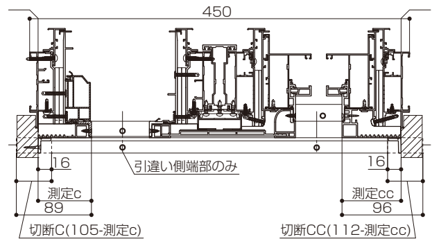
FIX窓—FIX窓連窓
