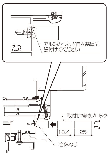
●上断面図
