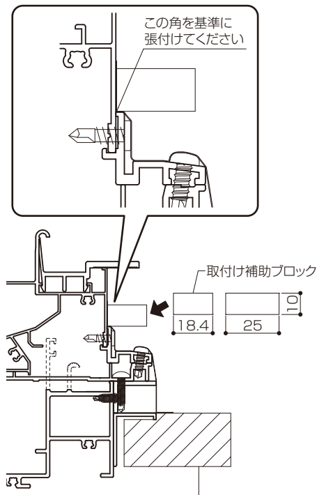
●下断面図
