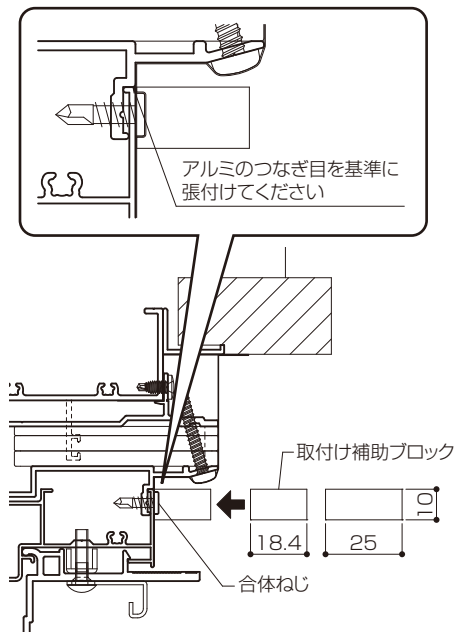
●上断面図
