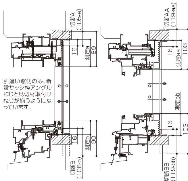
引違い側
