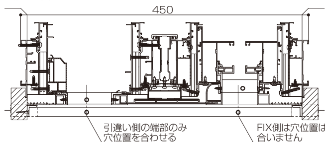
引違い側
