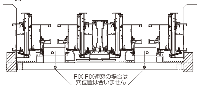
FIX側
