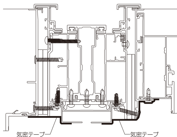
連窓方立カバー受け材の場合
