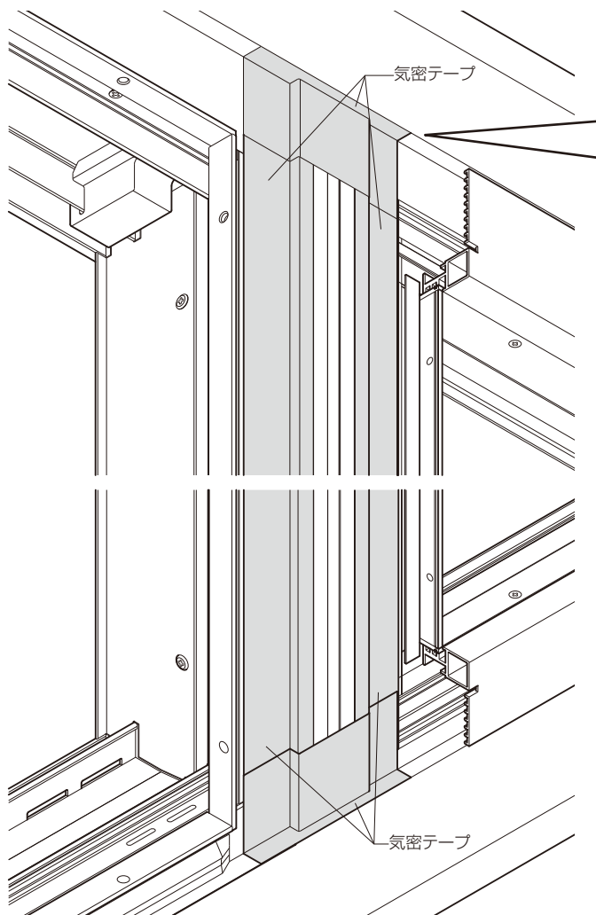
連窓方立カバー受け材の場合
