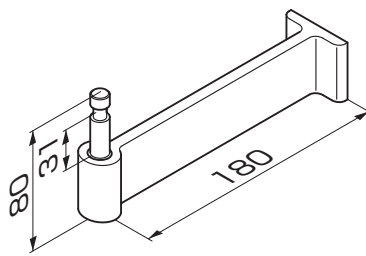
図1-3 VUS、VUW姿図
