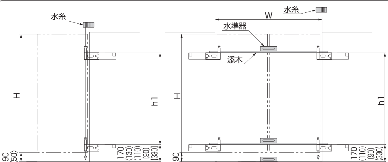
図1-1 施工寸法図
