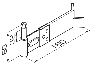
図1-2 AUS、AUW姿図
