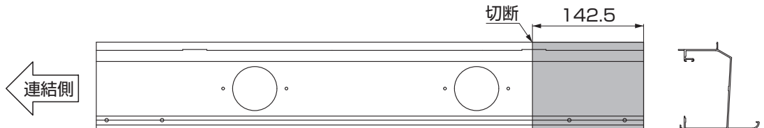
図4-2 前枠18延長
