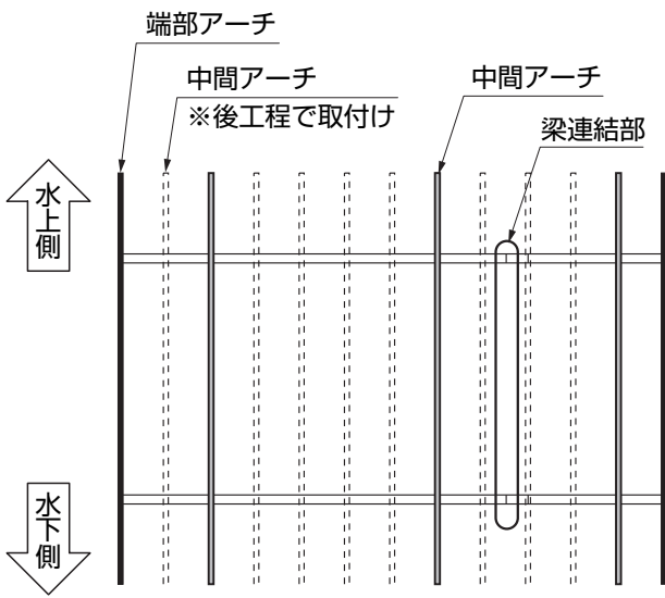
図3-1 18延長 (W54+W18)
