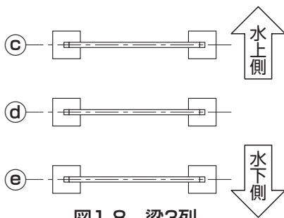
図1-8 梁3列
