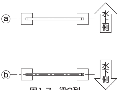
図1-7 梁2列
