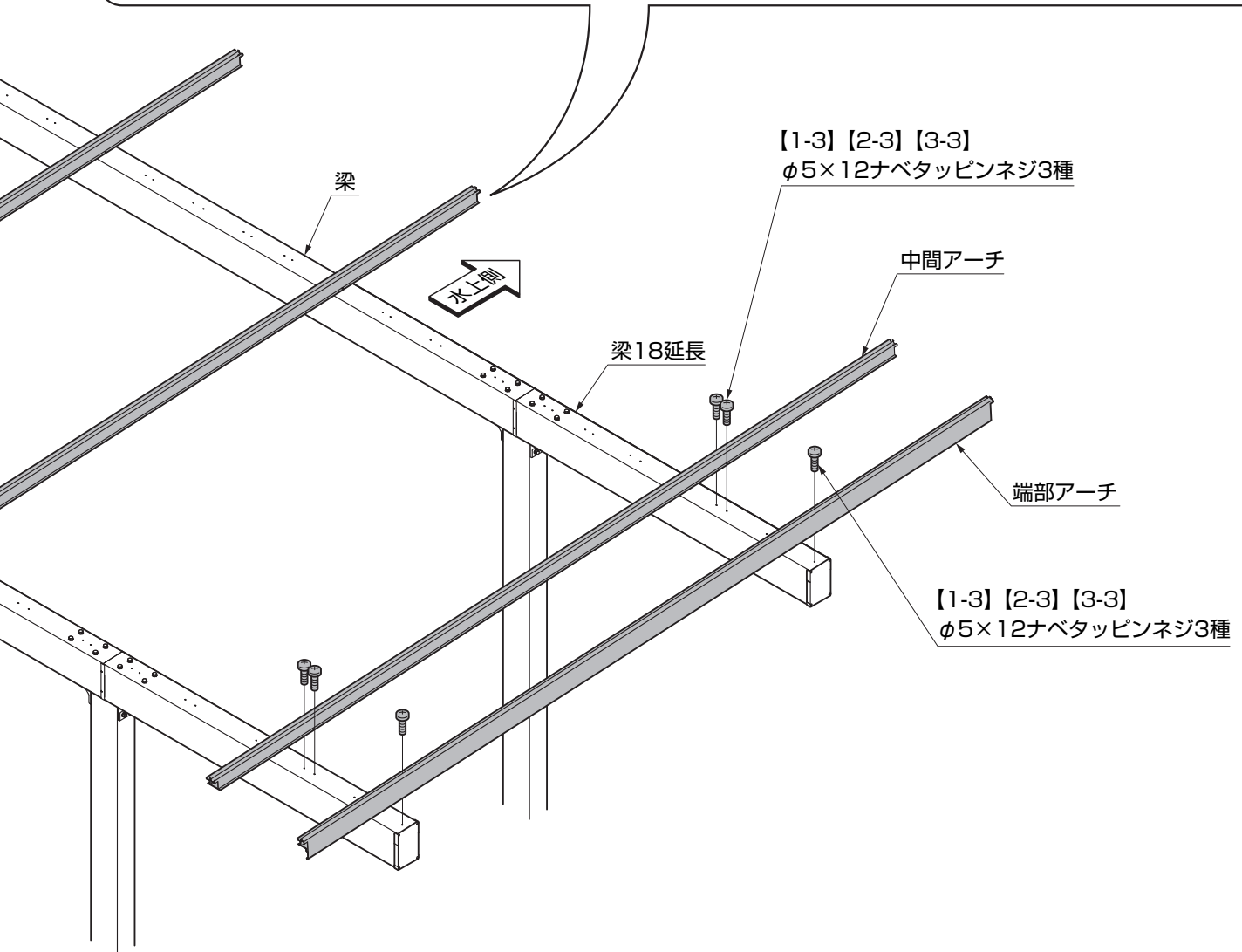
図3-2 18延長 (W60+W18)
