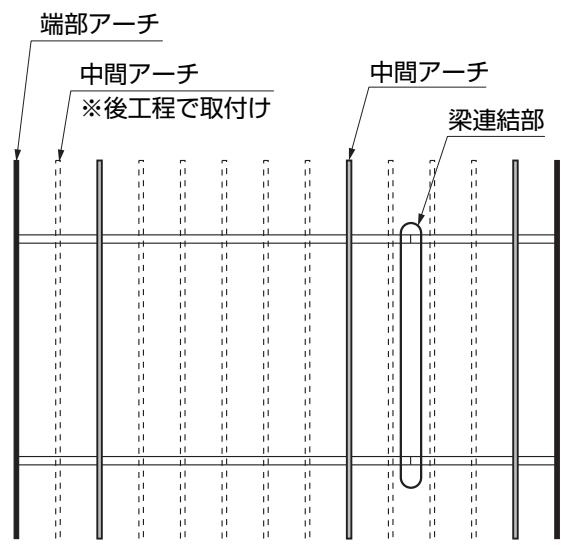
図3-2 18延長 (W60+W18)
