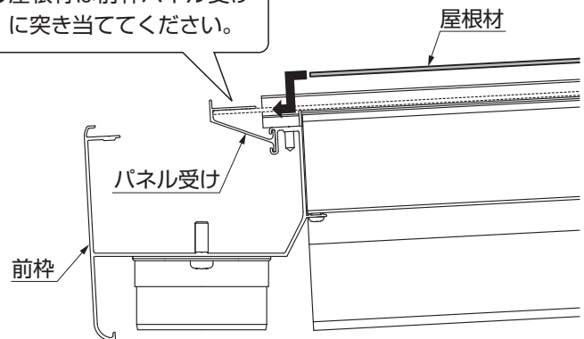
図6-4 前枠側
