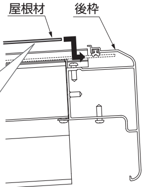
図6-3 後枠側
