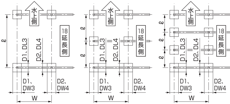
図1-1 4本柱
