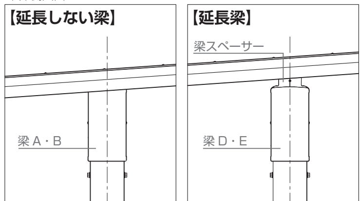
梁部側面図
