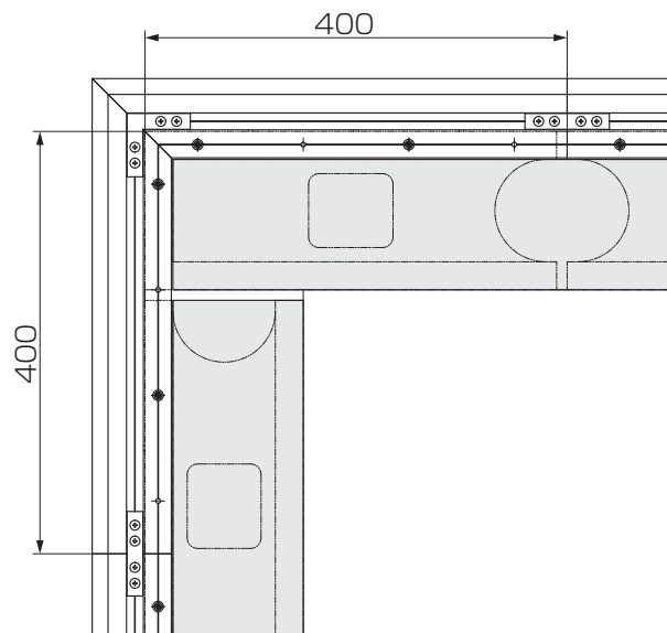
【出隅納まり】
