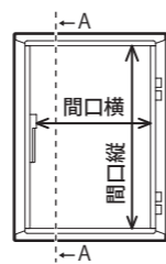
【扉開けた状態】
