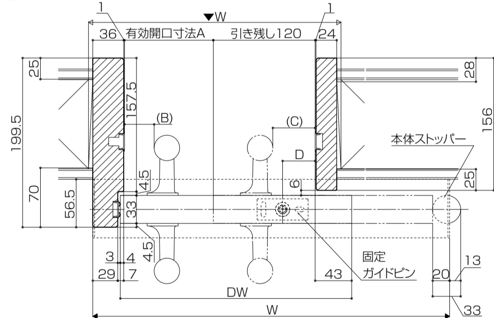
横断面図
