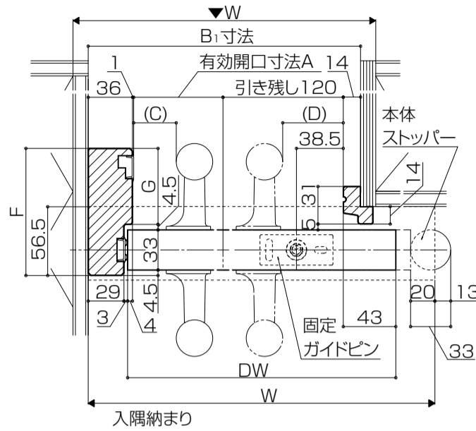
横断面図
