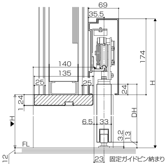
縦断面図
