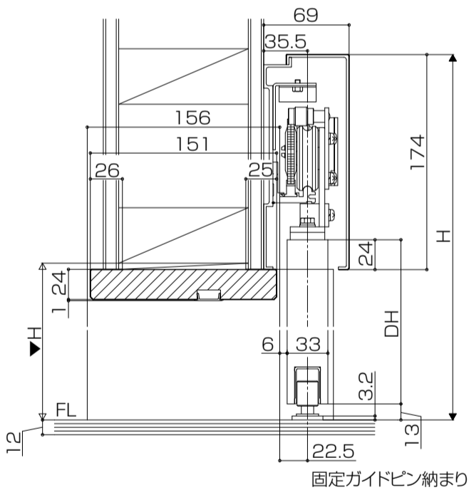
縦断面図
