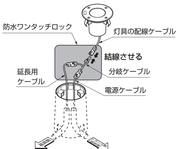
図3-4 複数灯設置の場合（コネクタの接続）
