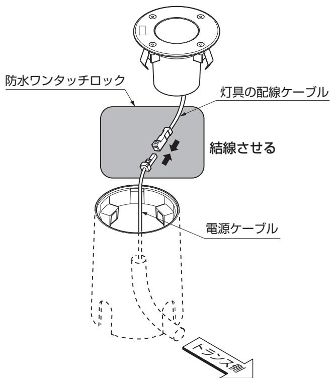
図3-3 単独設置の場合（コネクタの接続）
