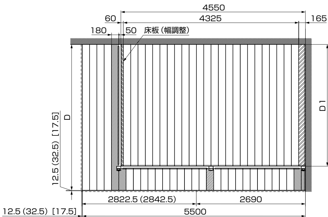
図2-4 デッキ割付図2.5間
