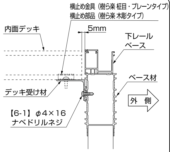
図1-13 側面図
