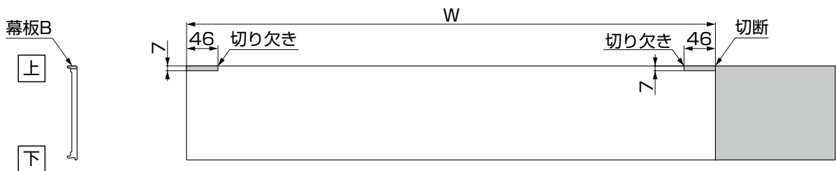
図2-2 間口用幕板の加工
