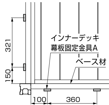
図2-3 取付けピッチ
