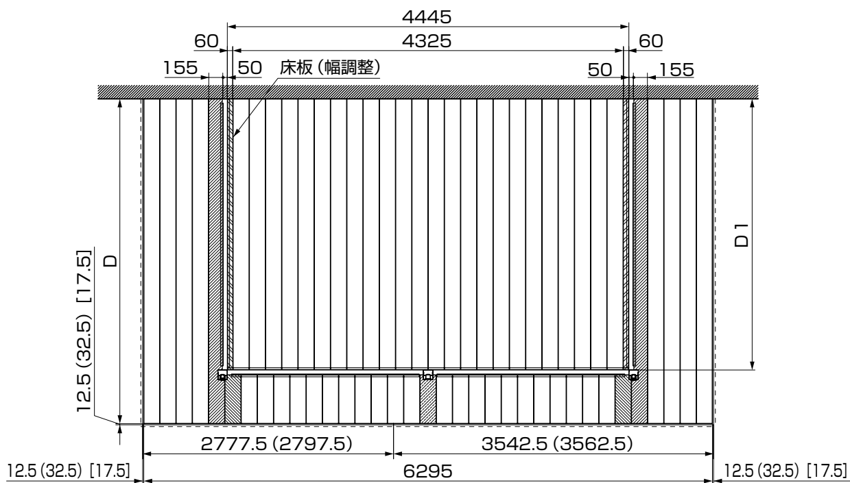
図1-4 デッキ割付図2.5間
