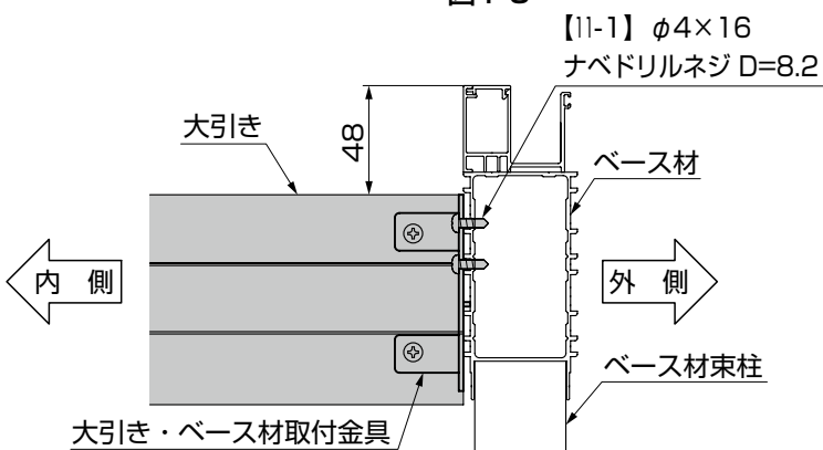
図1-7 正面図
