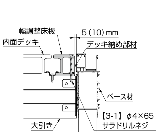
図1-19 基本仕様 デッキ納め部材を使用する場合
