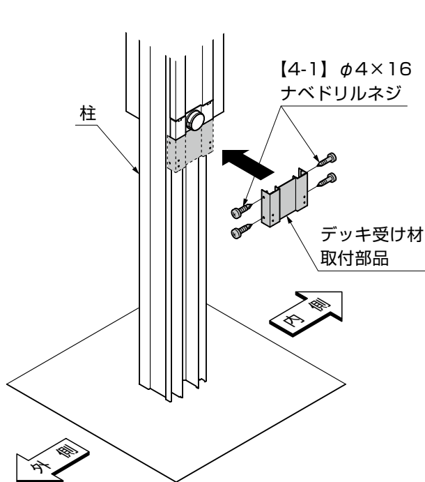
図4-9 基本仕様 主柱、中間柱、連棟柱の場合
