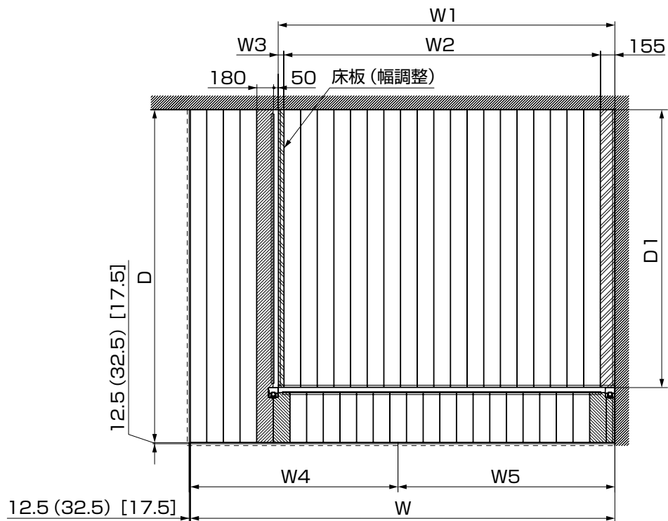
図2-2 デッキ割付図
