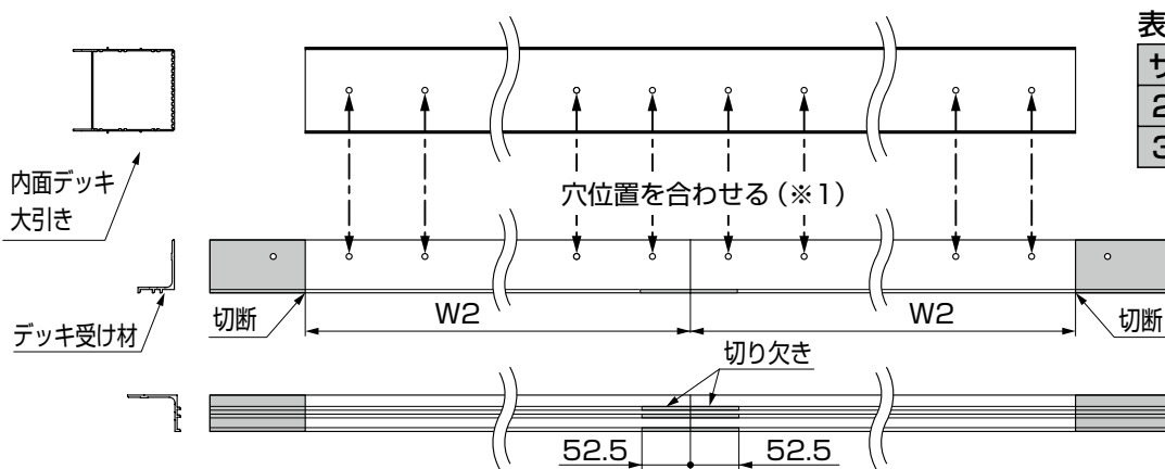
図1-11 2.5間、3.0間の場合
