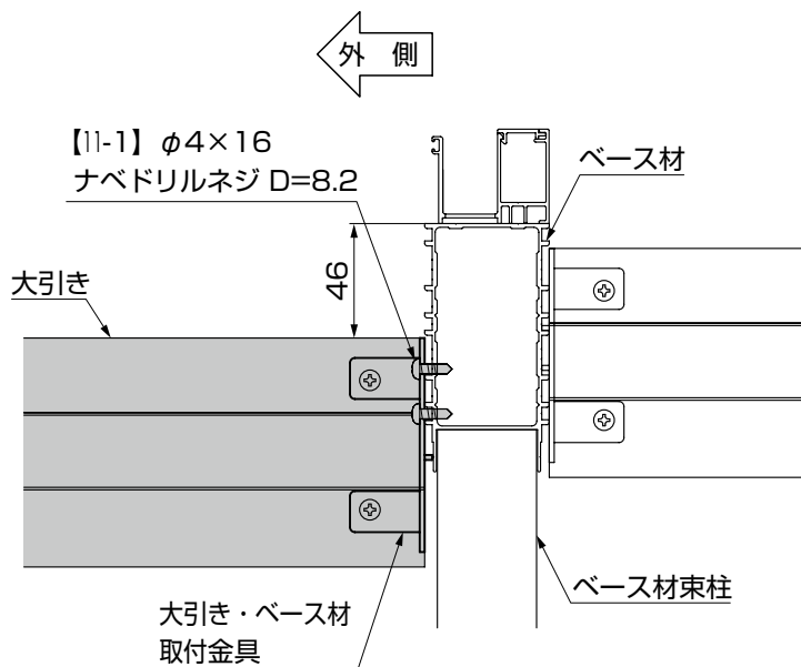
図4-4 正面図
