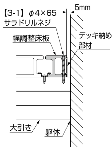
図1-21 入隅仕様
