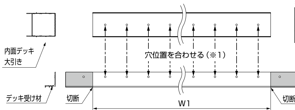
図1-10 1.5間、2.0間の場合
