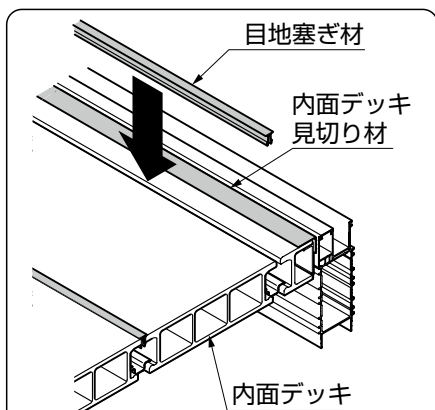
図1-23 基本タイプ
