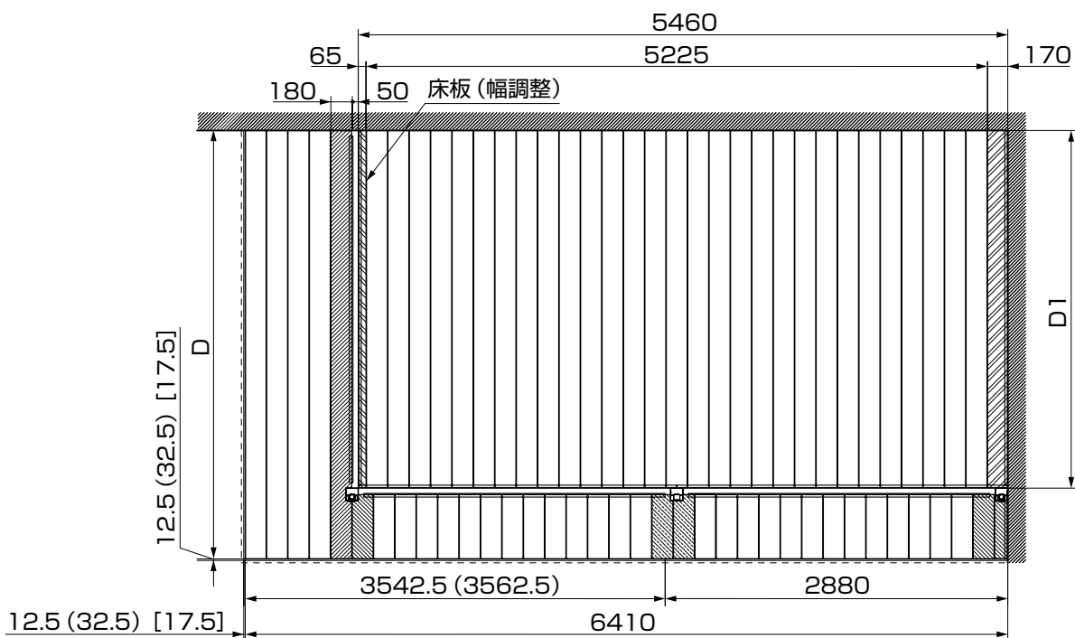
図2-5 デッキ割付図3.0間
