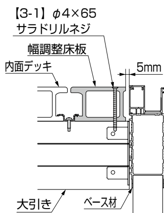
図1-20 基本仕様 床板直止めの場合
