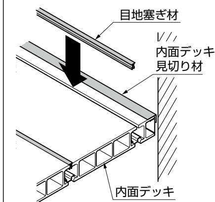
図1-24 入隅タイプ
