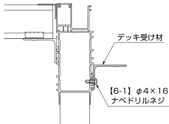
図4-7 側面図
