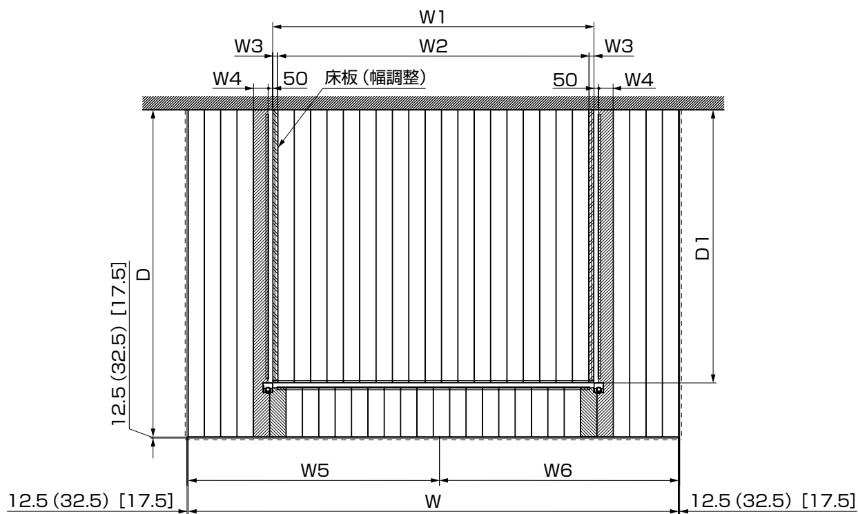
図1-2 デッキ割付図
