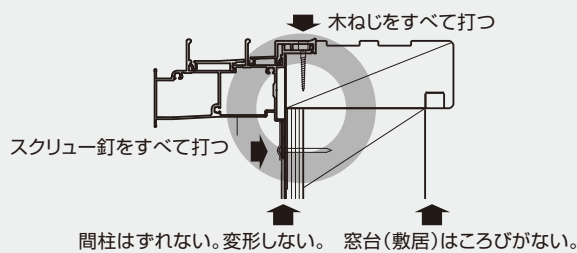
間柱はずれない。変形しない。窓台(敷居)はころびがない。
