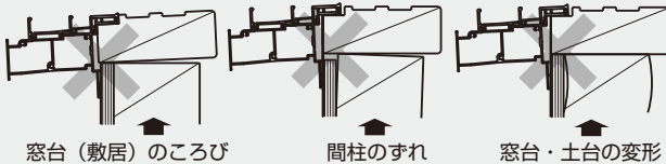
窓台(敷居)のころび
