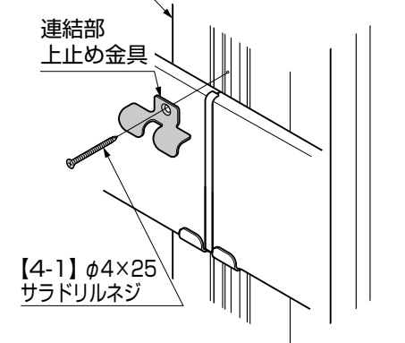
図1-6 連結部
