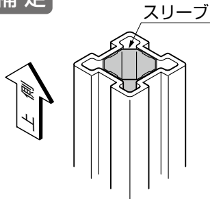
図1-1 T-08、T-10主柱
