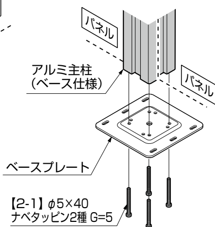
図2-2 側面固定の場合
