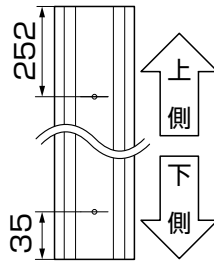
図1-2 T-12主柱
