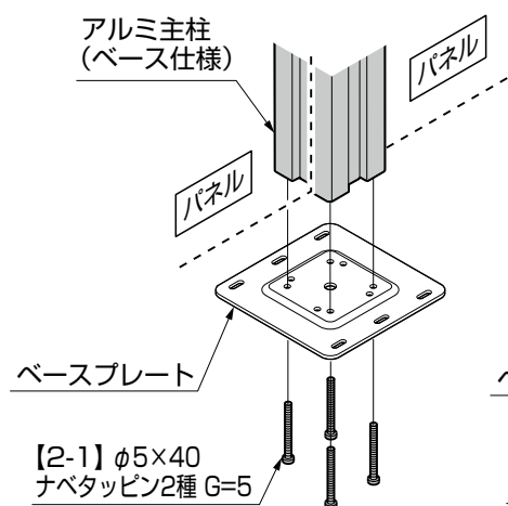
図2-1 正面固定の場合
