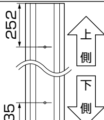
図1-2 T-12、T-18主柱
