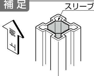
図1-1 T-08、T-10主柱
