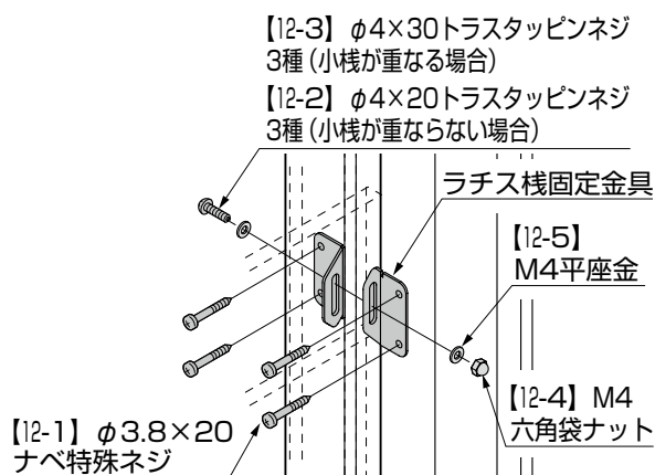
図2-8 T-18の場合
