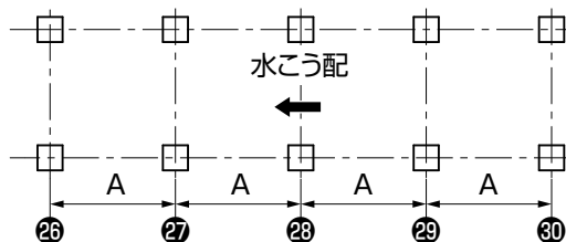
図1-6 8本柱+12延長
