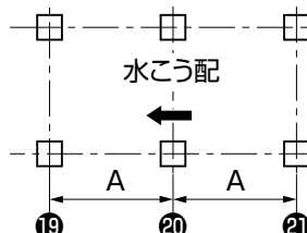
図1-4 4本柱+12延長
