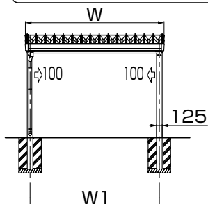
図2-1 間口30・36サイズ
