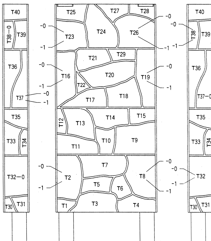
背面図
