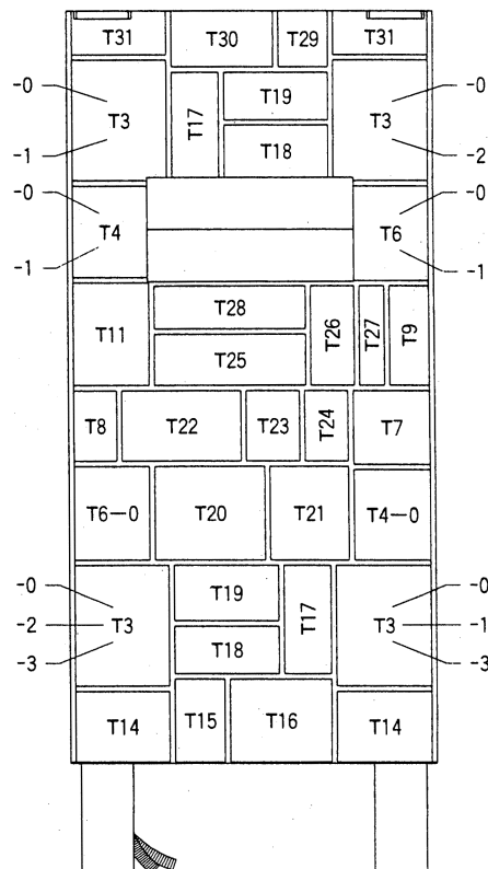
背面図
