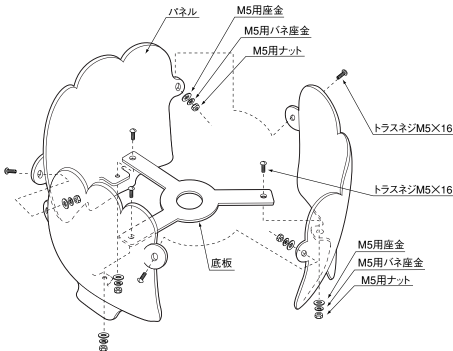
梱包明細 プランターカバーBタイプ
