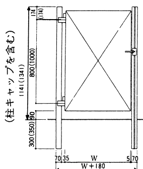
〔片開き〕
