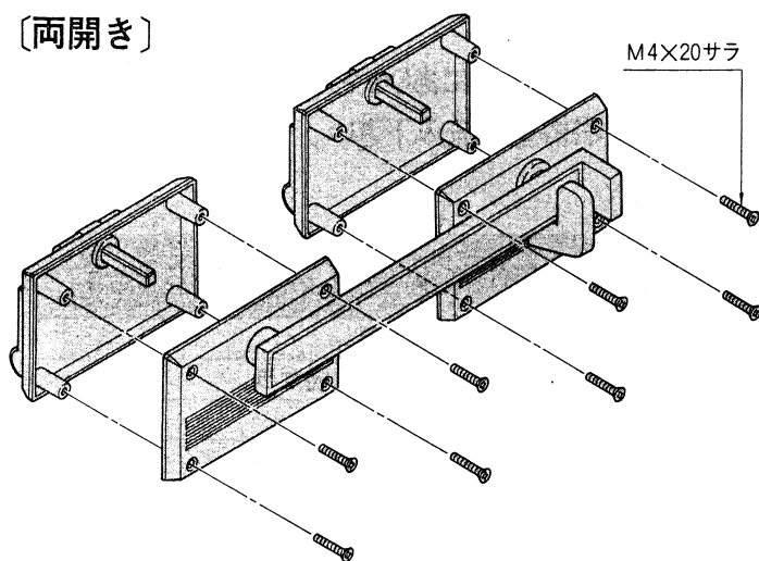
〔錠取付詳細図〕 〔両開き〕
