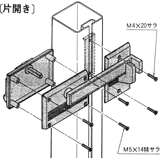
〔片開き〕
