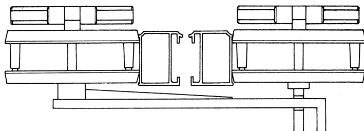
〔錠取付詳細図〕 〔両開き〕
