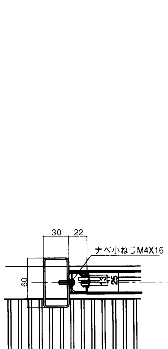
B-B断面図
