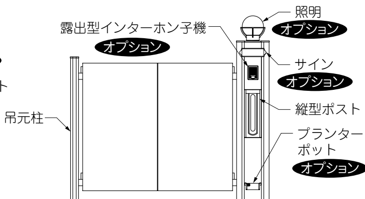
図2-4 ショートポール両柱+門柱仕様
