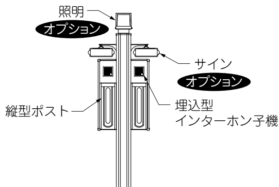
図2-2 2世帯専用ポール仕様
