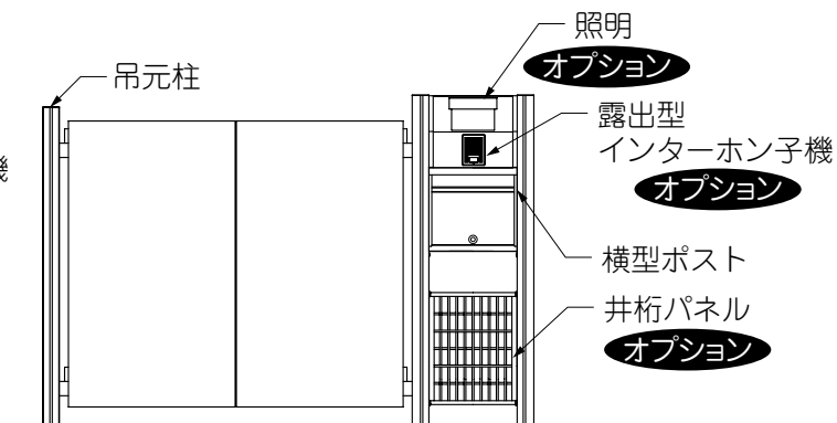
図2-6 門柱仕様
