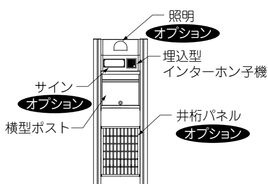
図2-5 単独仕様
