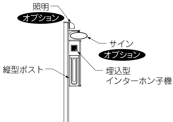
図2-1 ショートポール片柱仕様
