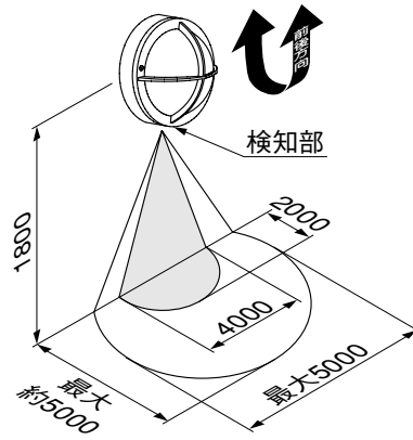
図1-3 前後検知範囲の目安
