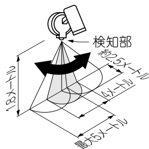
左右検知範囲の目安
