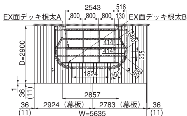
(2) デッキ根太伏図
