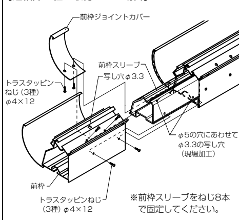
【連結部に柱が取付かない場合】
