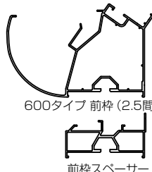
前枠スペーサー
