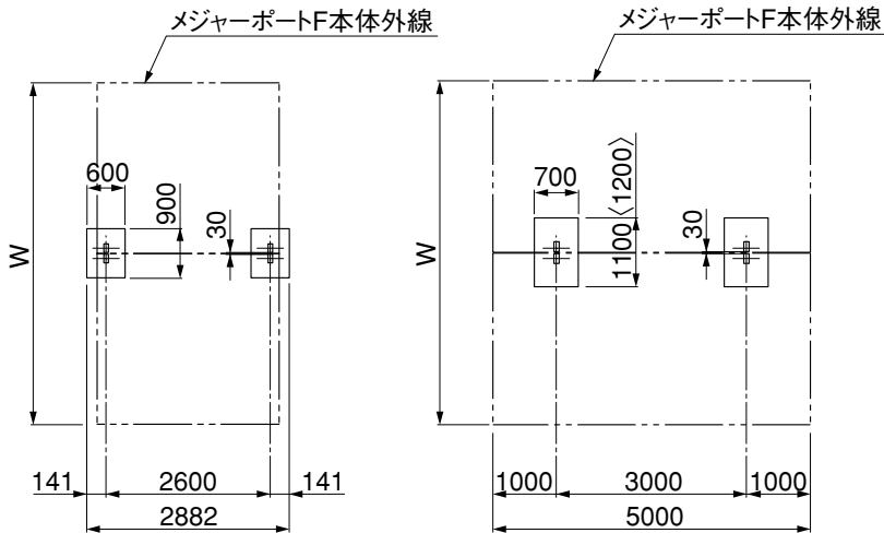
図1-1 29サイズ
