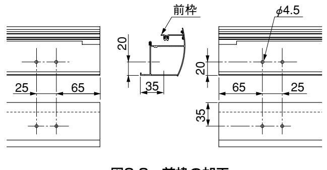
図2-2 前枠の加工
