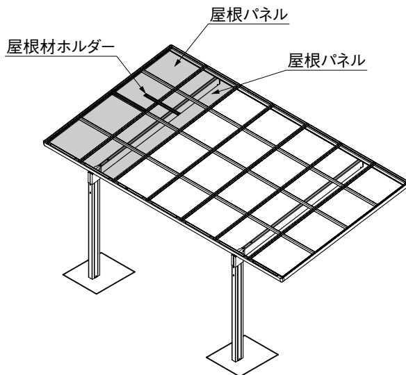
図5-3 屋根材ホルダーの取付け
