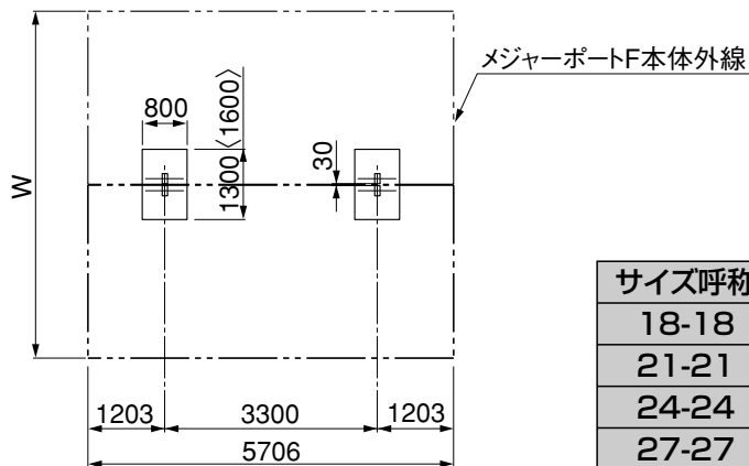
図1-3 57サイズ
