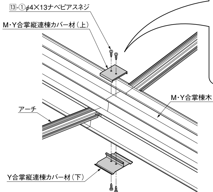
図3-2 Y合掌縦連棟
