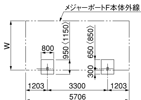
図1-3 57サイズ
