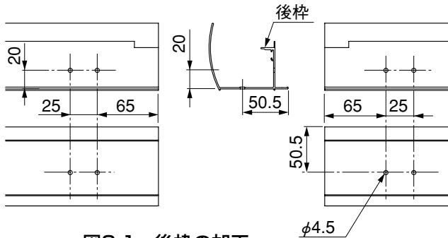
図2-1 後枠の加工
