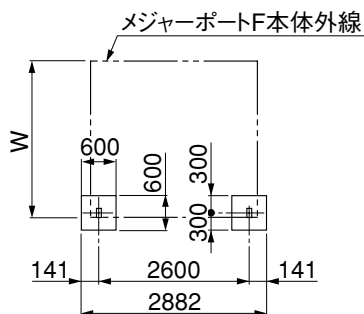
図1-1 29サイズ
