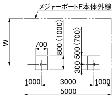
図1-2 50サイズ
