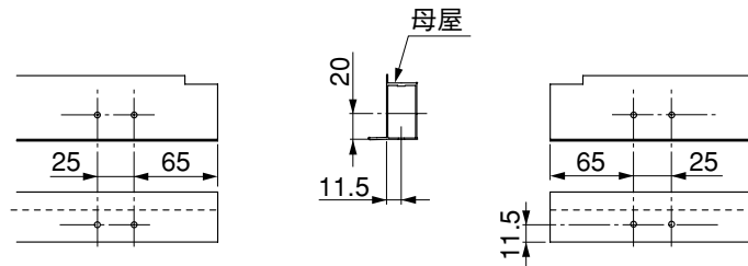
図2-3 母屋の加工
