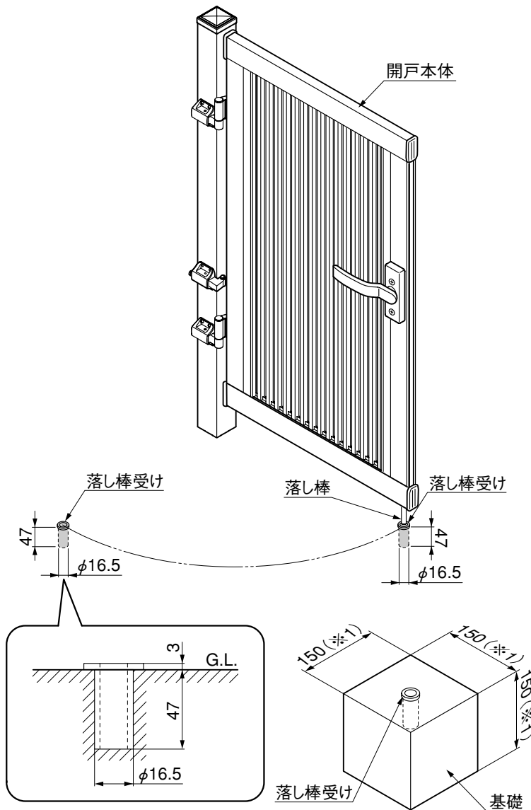
図9-1 基礎寸法
