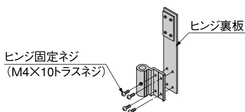
図2-1 左勝手のヒンジ組替え
