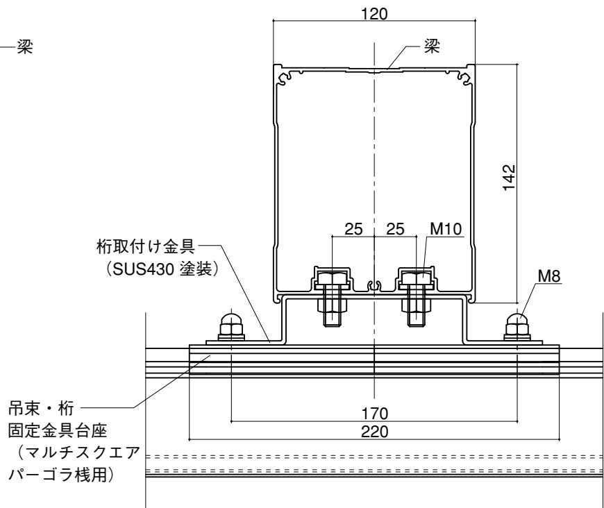
A-A 縦断面図
