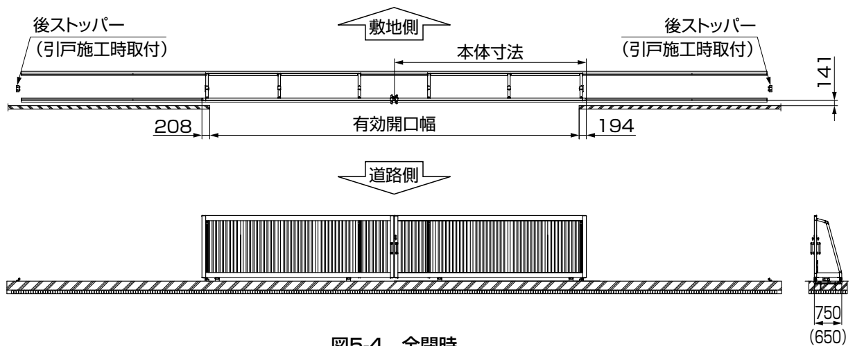
図5-4 全閉時
