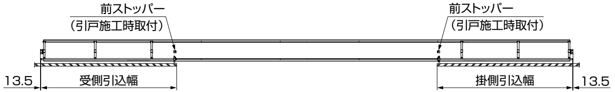
図5-3 全開時
