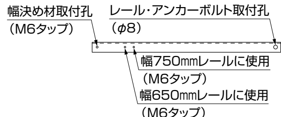
図4-3 位置決め材2
