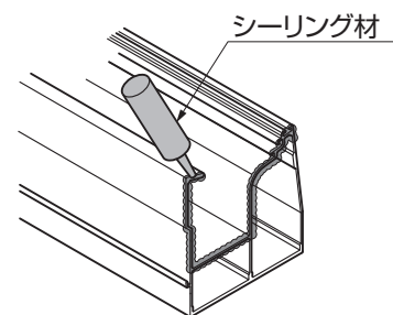
図1-3 桁のシーリング箇所
