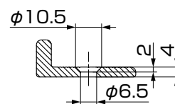
図10-13 φ6.5サラ孔断面図
