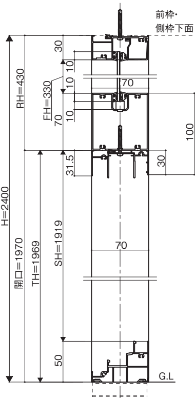
・テラスサッシ納まり
