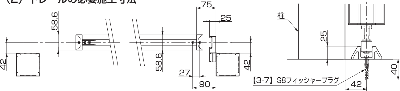
図4-1 柱（端部用）側
