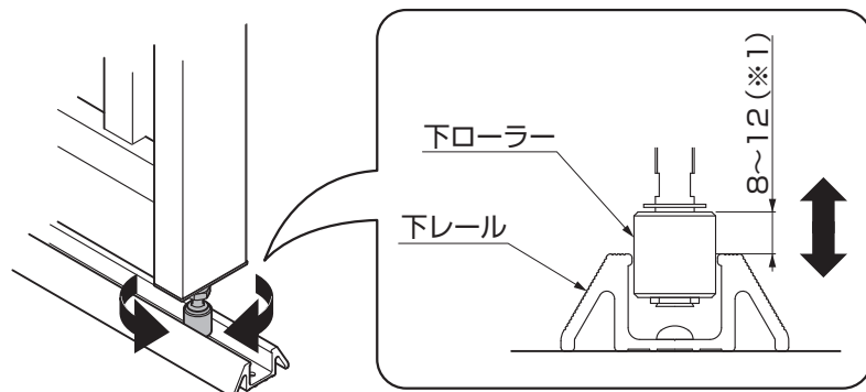
図10-7 下ローラーの長さ調整
