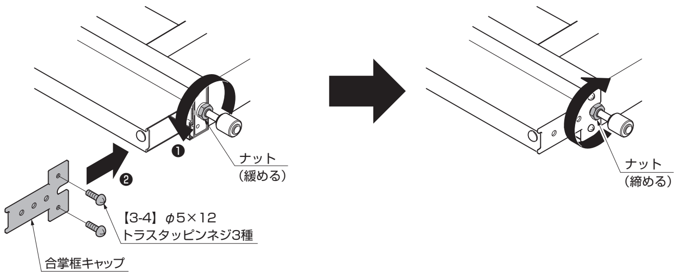
図10-3 合掌框キャップの取付け
