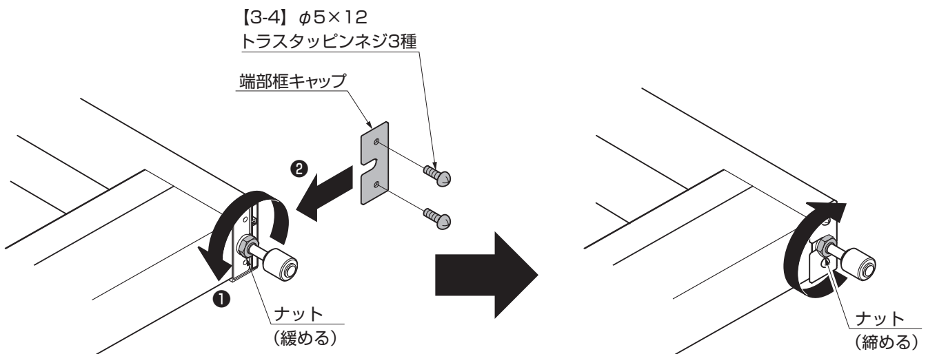
図10-4 端部框キャップの取付け
