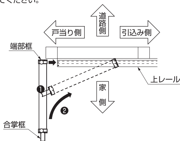
図10-5 上ローラーの吊込み
