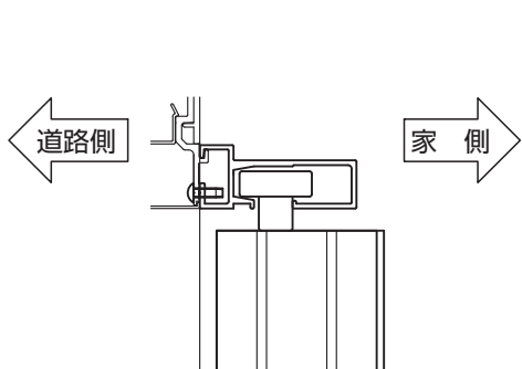
図10-6 道路側・家側方向
