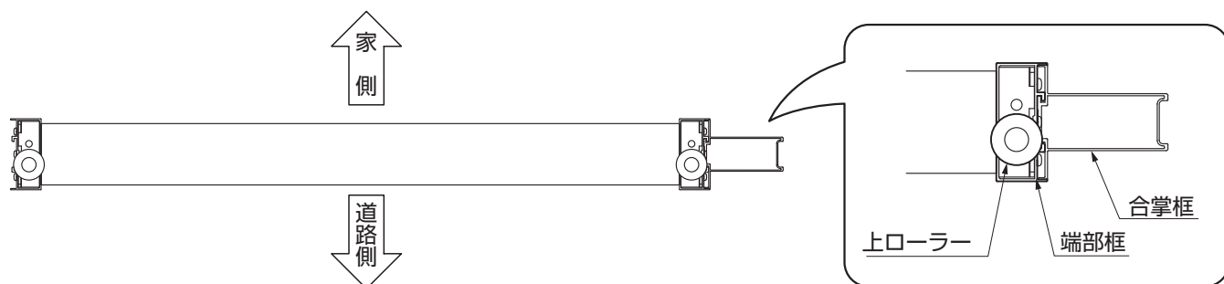
図10-2 合掌框の取付け方向(左引き) ※右引きの場合は左右対称
