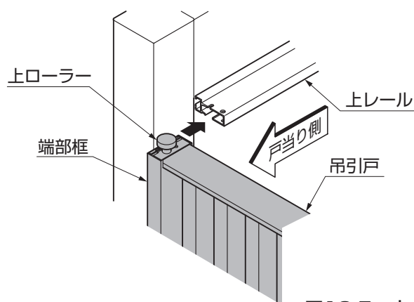
図10-5 上ローラーの吊込み
