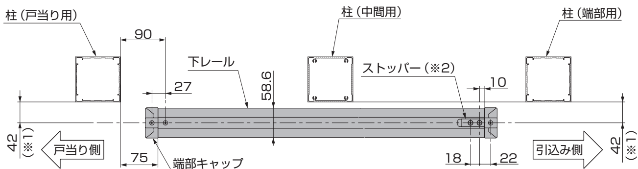
図7-1 下レール取付け位置
