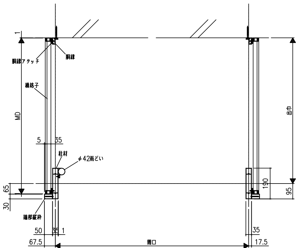
Z1-Z1断面図：下部納まり図
