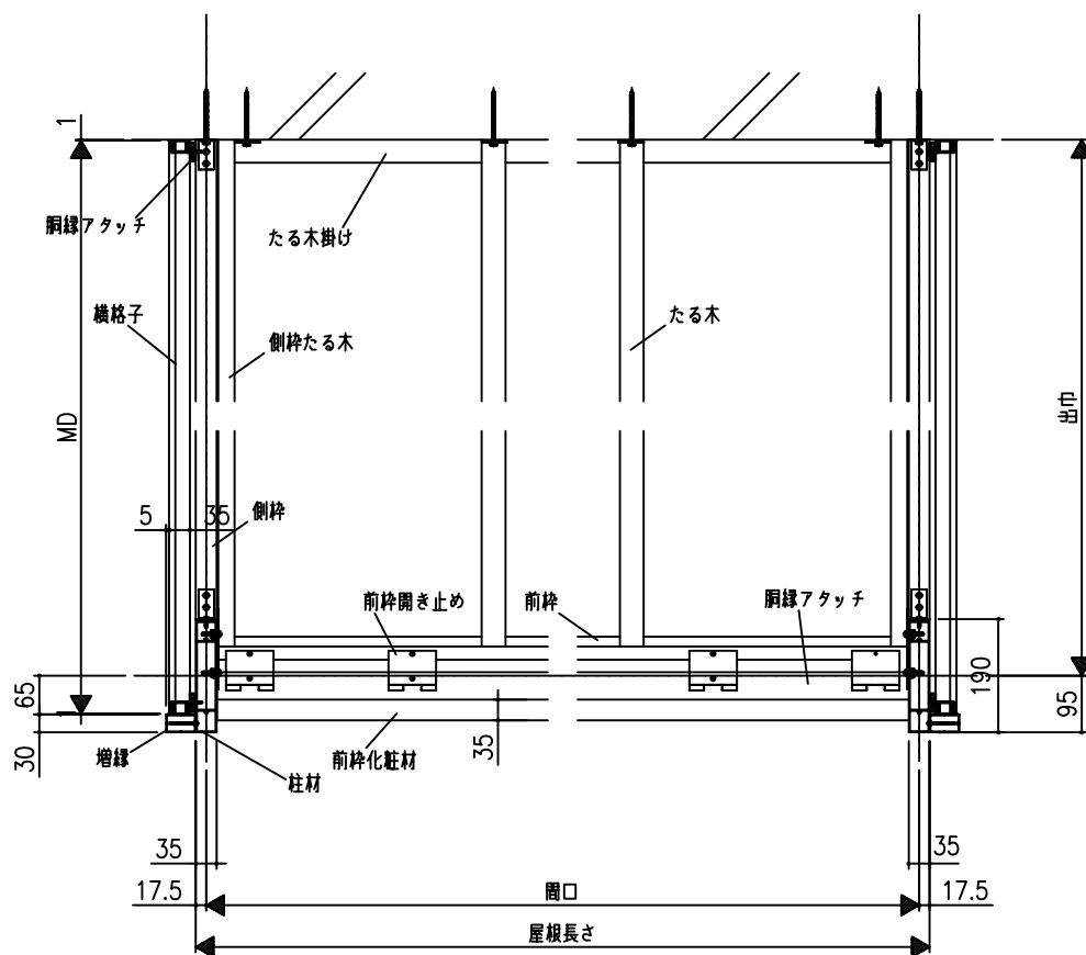
Z2-Z2断面図：上部納まり図
