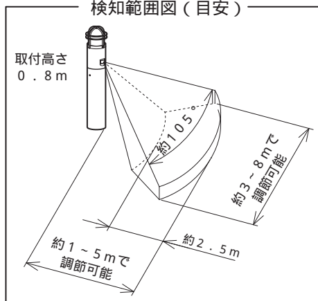
検知範囲図（目安）
