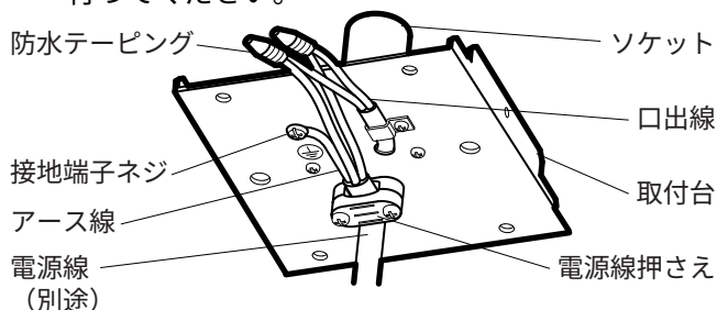
電源線押さえの使い方
