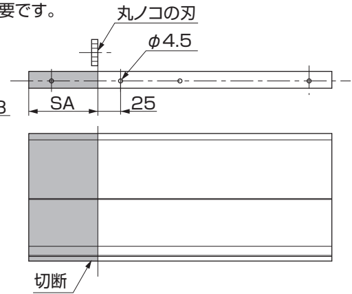
図2-9 側枠カバー加工図
