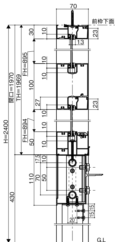
・FIX納まり
