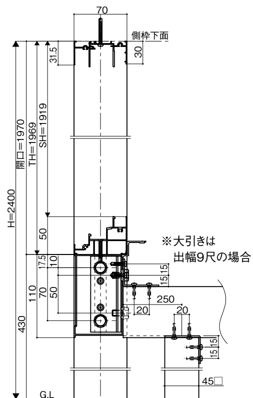
・テラスサッシ納まり
