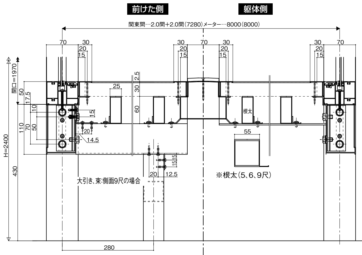
・FIX納まり
