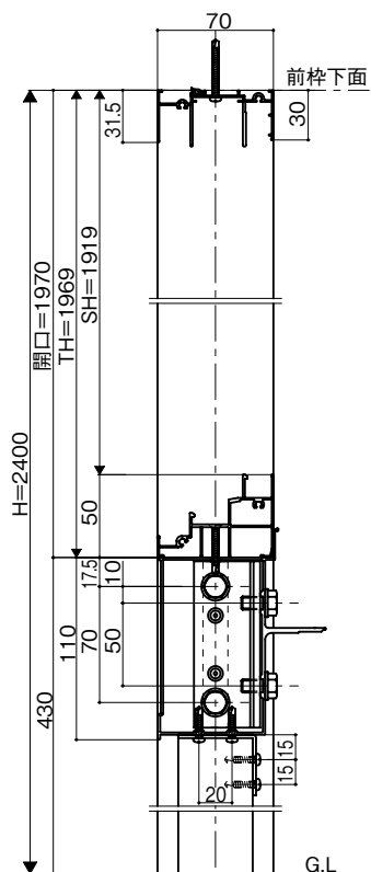
・テラスサッシ納まり
