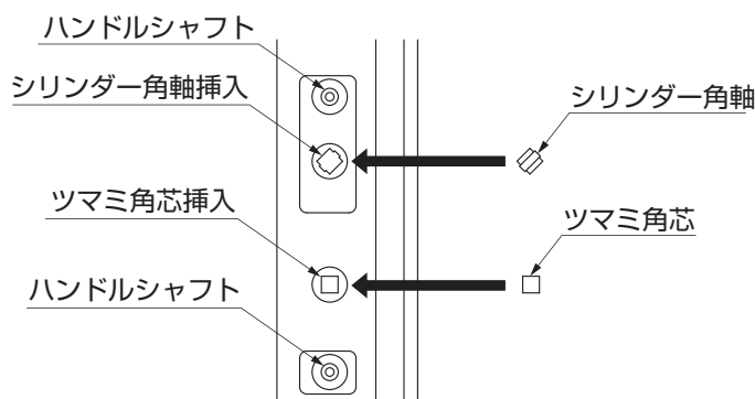
図6-12 シリンダー角軸、つまみ角芯挿入向き
