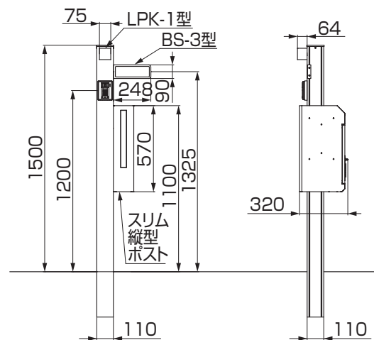
照明: LPK-1型、サイン: BS-3型、ポスト: スリム縦型ポスト
