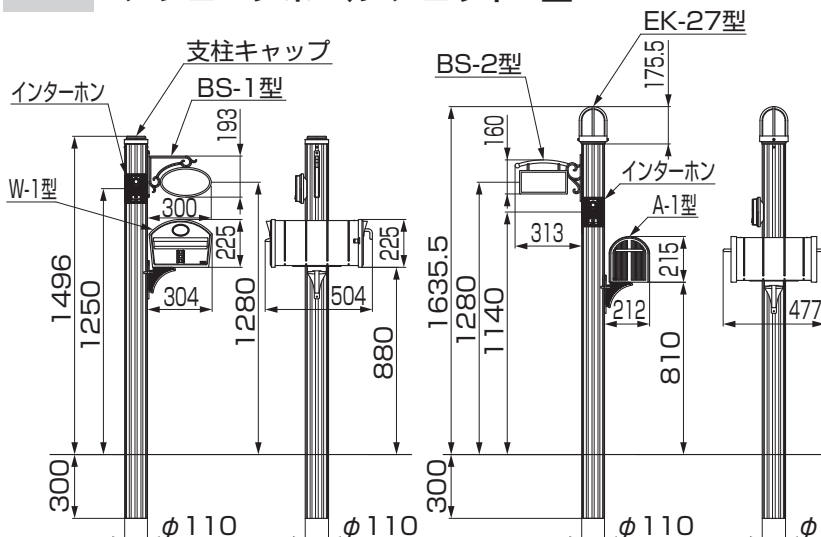
支柱キャップ、サイン: BS-1型、ポスト: W-1型
