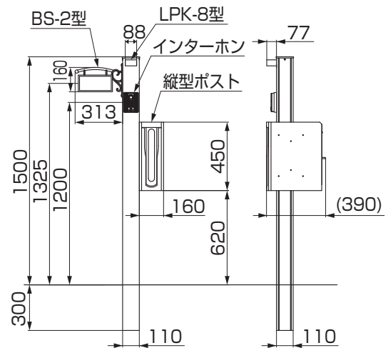
照明: LPK-8型、サイン: BS-2型、ポスト: 縦型ポスト
