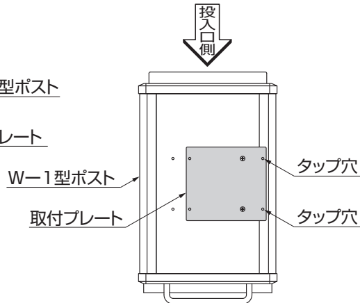
図3-2 外観左側に横付けする場合
