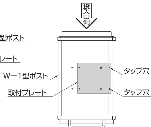
図3-8 外観左側に横付けする場合
