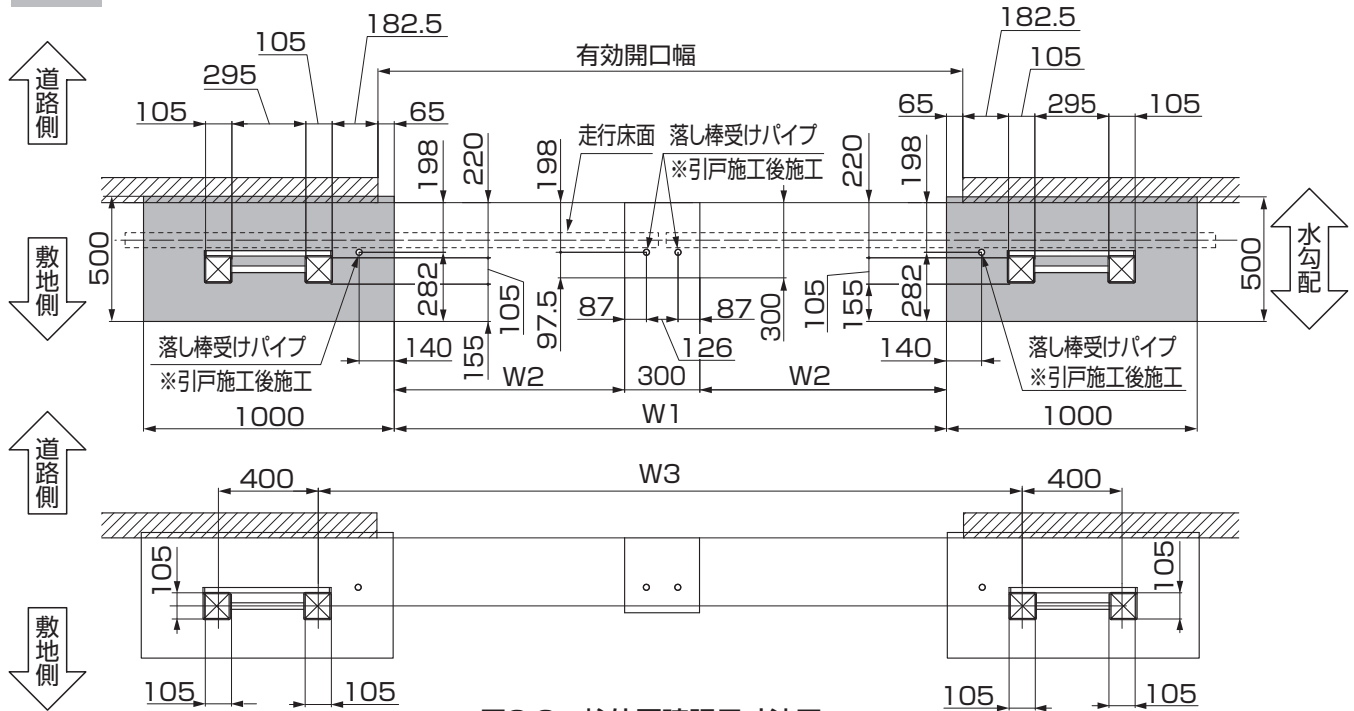
図2-2 柱位置確認用寸法図
