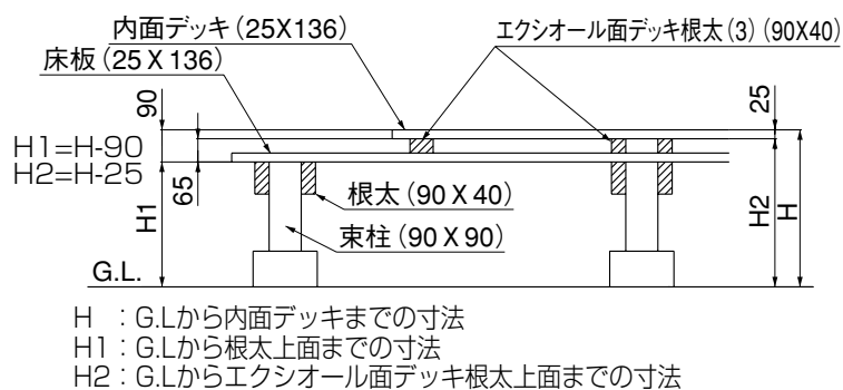
内面デッキ仕様
