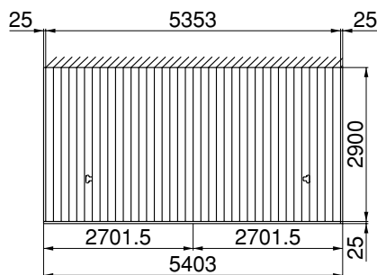
フラットデッキ仕様
