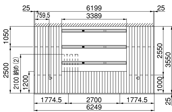
内面デッキ仕様
