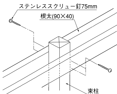
内面デッキ仕様の内面デッキ貼付け範囲の場合
