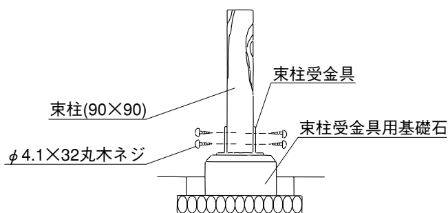
埋込み式（束柱受金具使用）
