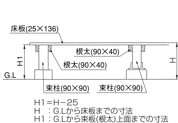
フラットデッキ仕様
