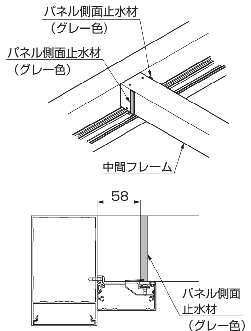
図8-4 B部詳細図
