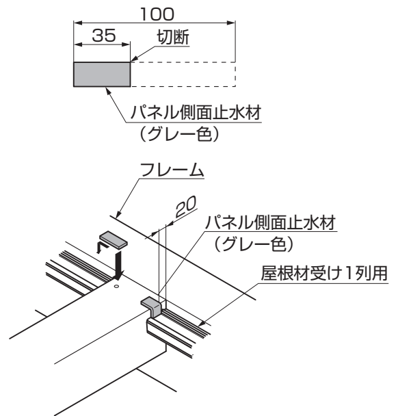
図8-2 A部詳細図
