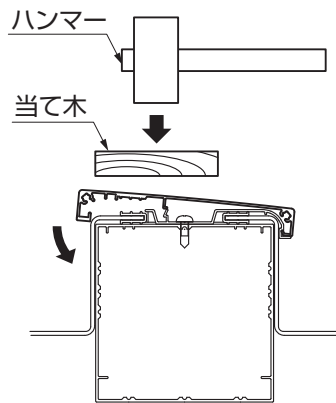
図9-38 中間部の場合
