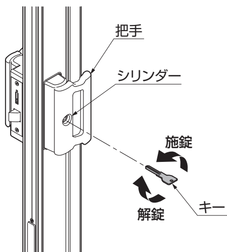
図3-1 シリンダーが右側にある場合
