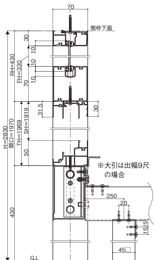
・テラスサッシ納まり
