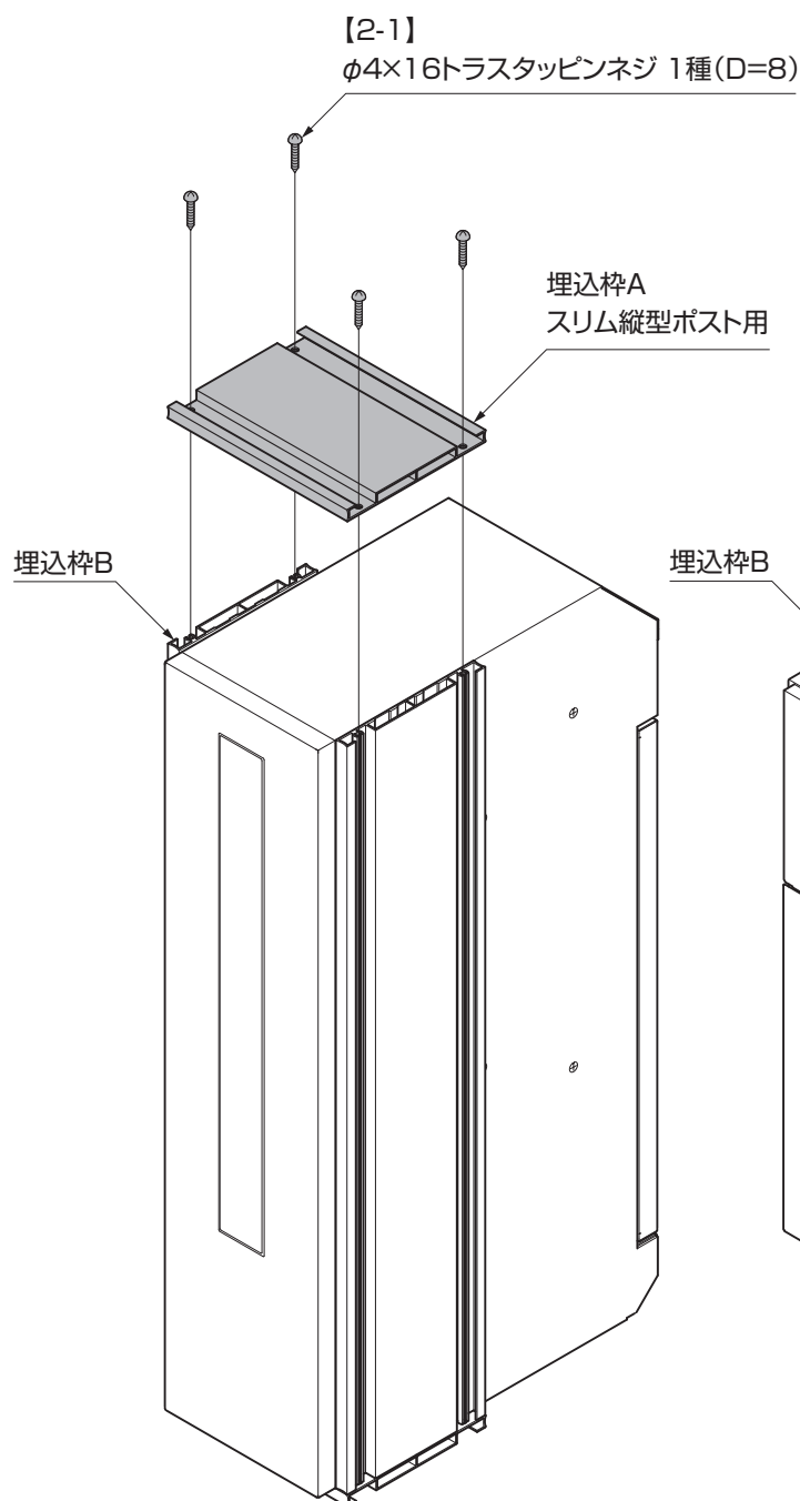
図2-5 スリム縦型ポスト
