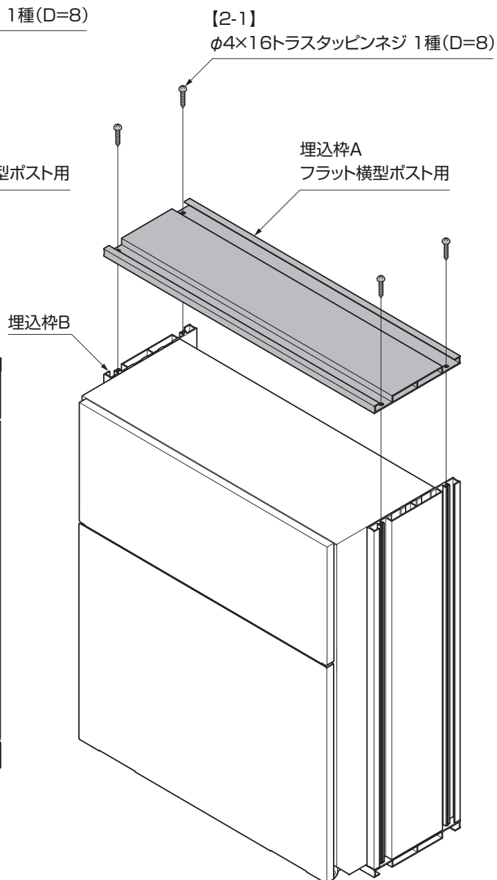
図2-6 フラット横型ポスト
