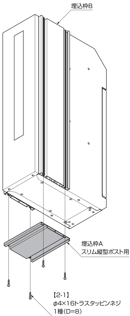
図2-3 スリム縦型ポスト
