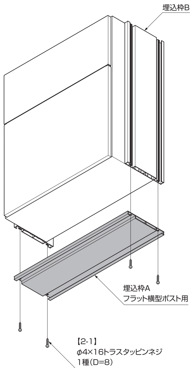
図2-4 フラット横型ポスト
