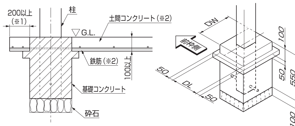
図1-7 土間コンクリート併用基礎の納まり
