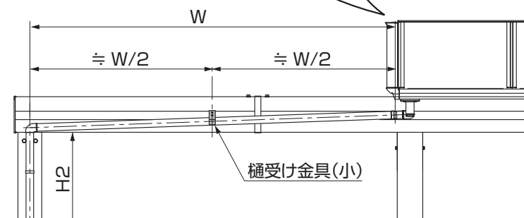
図3-8 W70の場合 でんでん・樋受け金具取付け位置
