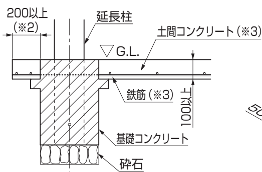
図1-5 土間コンクリート併用基礎の納まり
