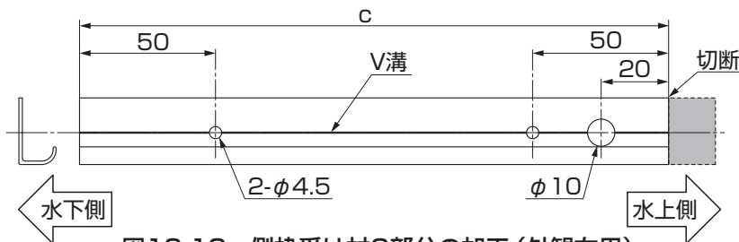
図10-13 側枠受け材C部分の加工（外観右用）
