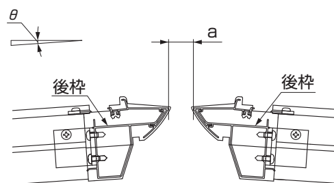
図2-8 B部詳細図
