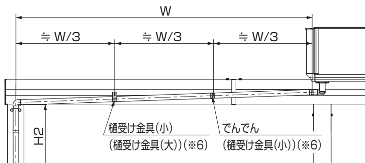
図3-9 W80の場合 でんでん・樋受け金具取付け位置
