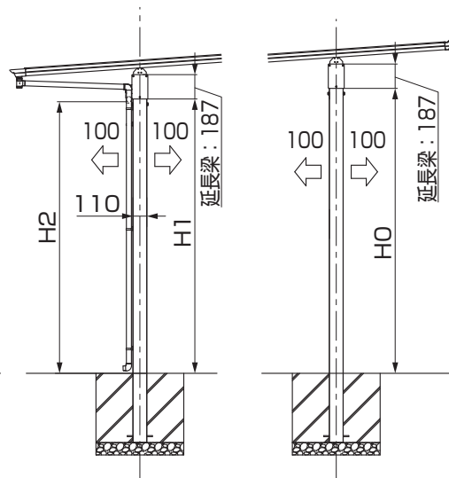
図2-2 水下延長の場合
