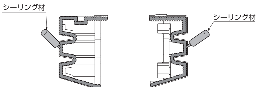
図10-19 前枠コーナーキャップ シーリング箇所
