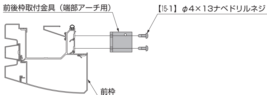
図5-3 プレミアムワイド用
