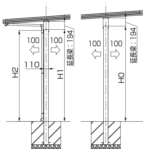
図2-5 水下延長の場合
