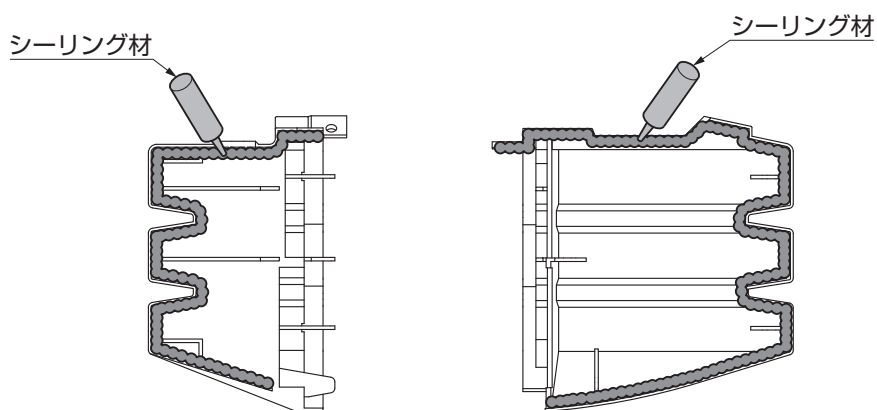
図10-20 後枠コーナーキャップ シーリング箇所
