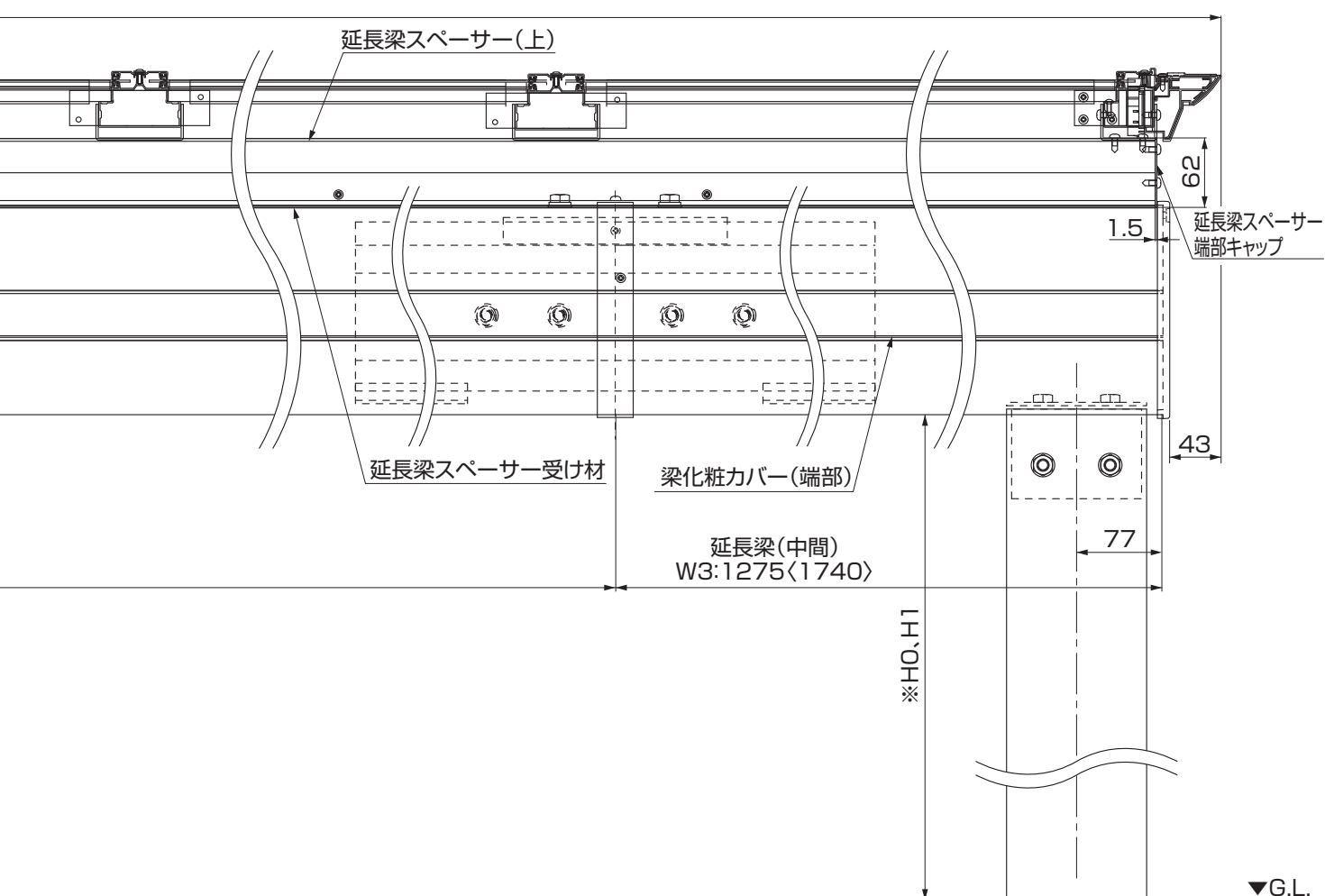
図3-2 プレミアムワイド延長梁
