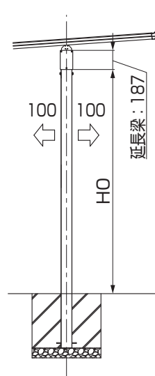
図2-3 水上延長の場合
