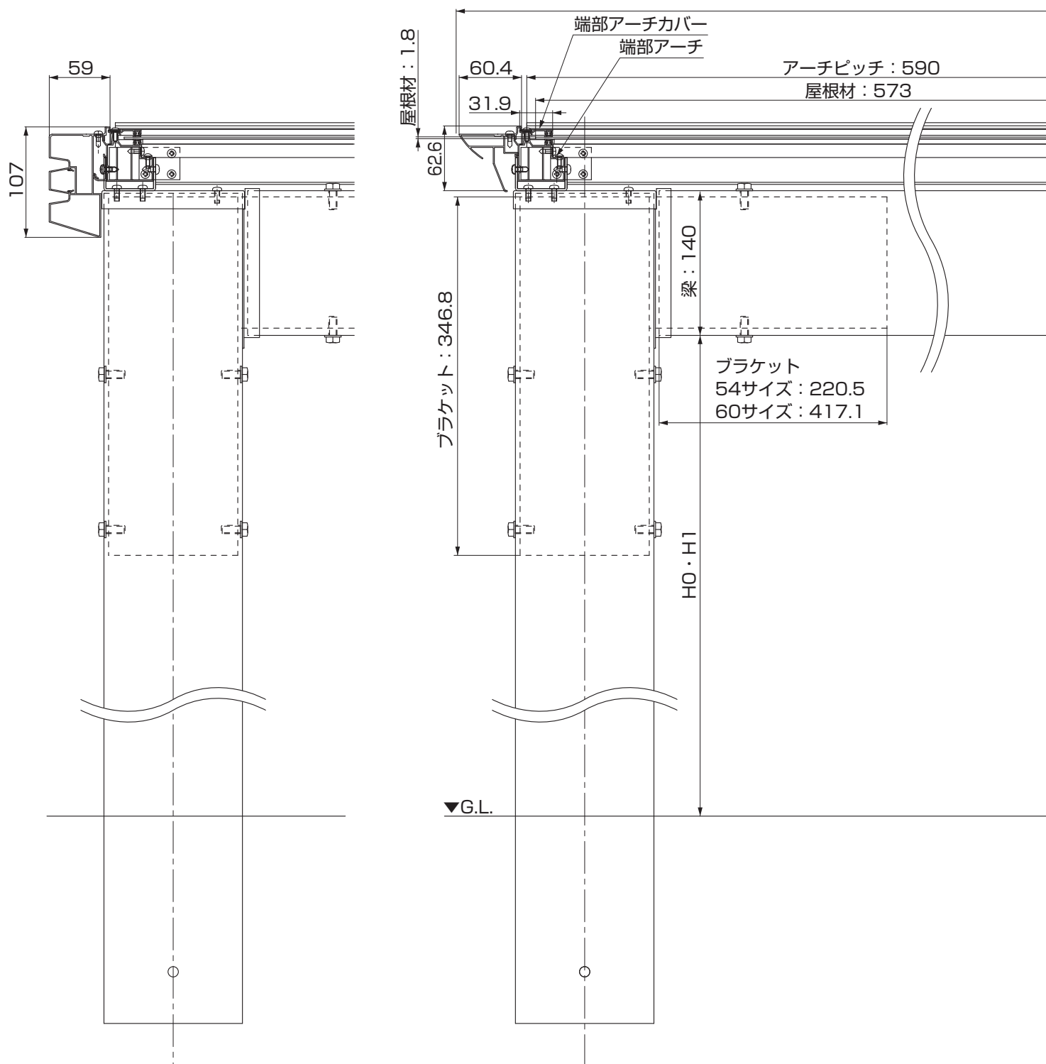
図1-2 プレミアムワイド
