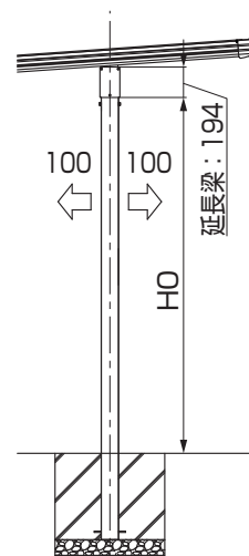
図2-6 水上延長の場合
