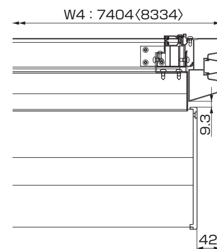
図3-2 プレミアムワイド延長梁
