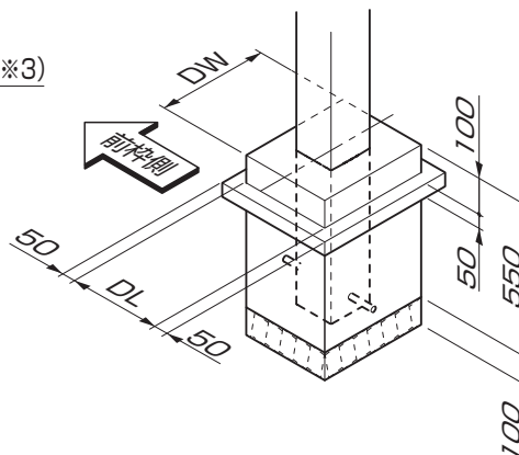
図1-5 土間コンクリート併用基礎の納まり
