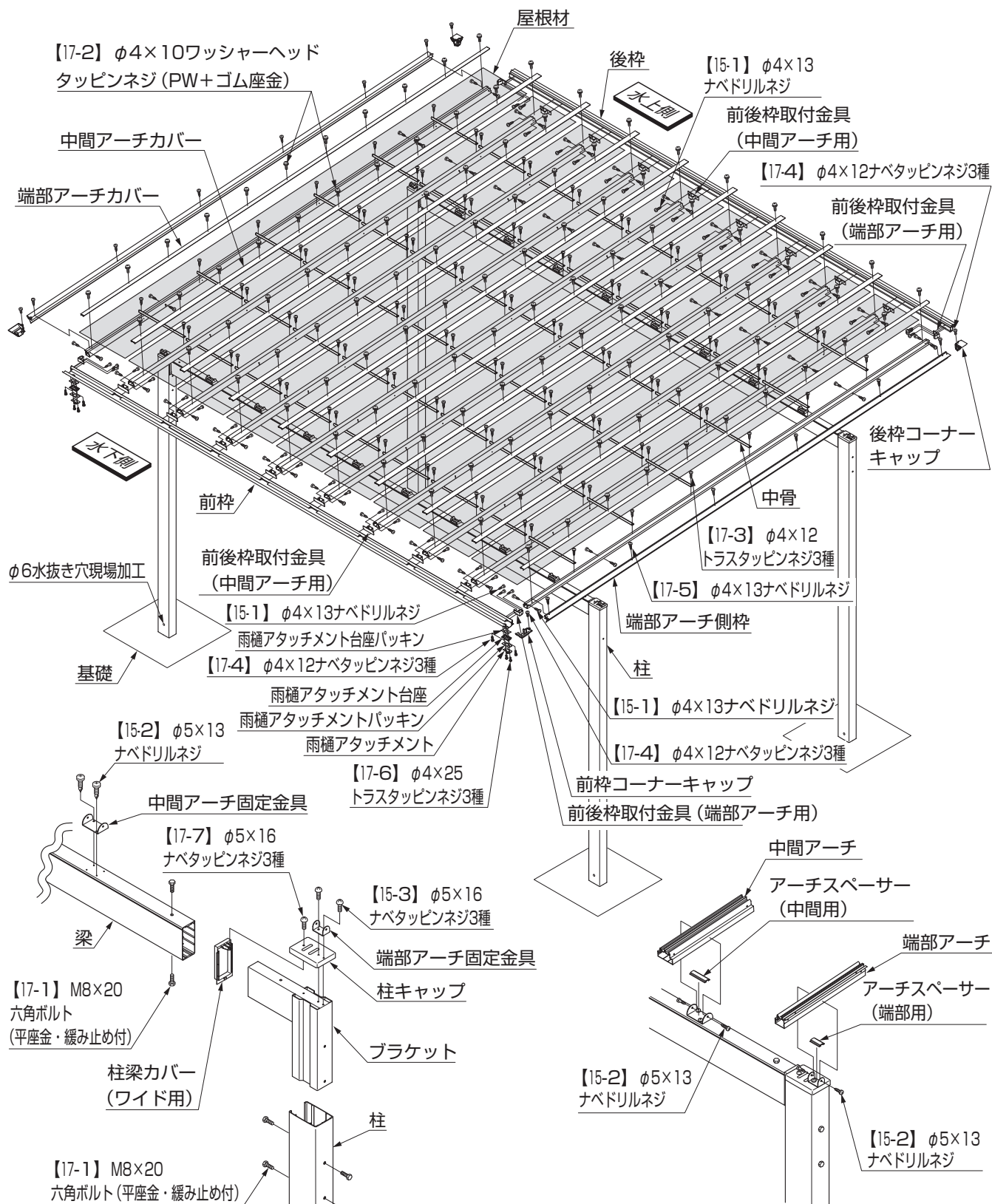
図1-1 柱梁取付詳細
